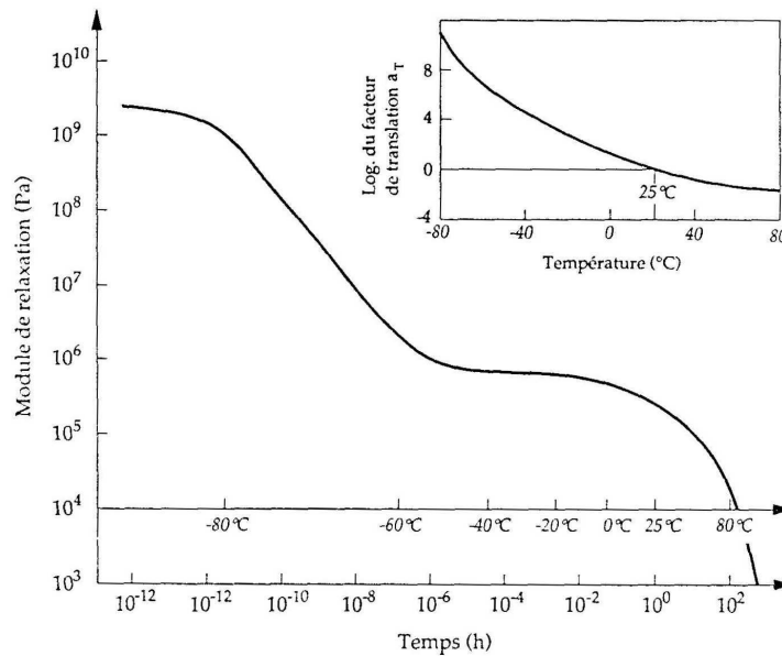
Figure I- 21 : Courbe maîtresse obtenue à partir des données précédentes. En encart, variation du facteur de translation en fonction de la température (Oudet 1994).
