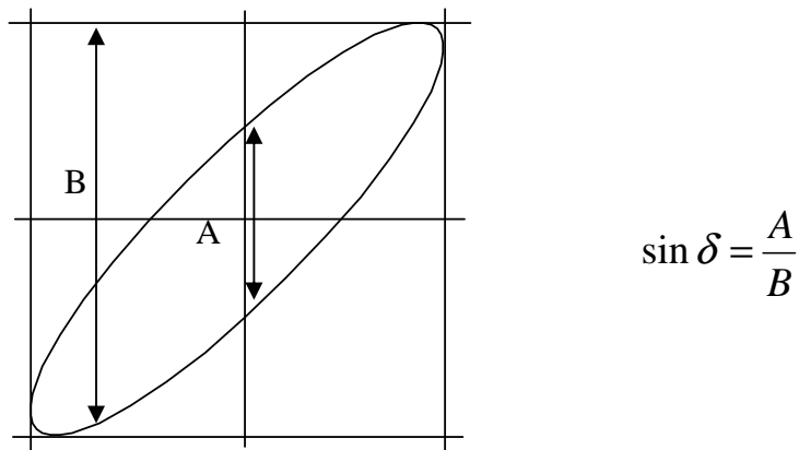
Figure III- 13 : Détermination du déphasage par la méthode de Lissajous
