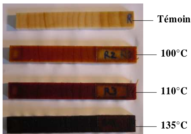
Figure V- 48 : Aspect des échantillons d’Epicéa de la direction radiale, saturés en eau, après traitement à différentes températures pendant une vingtaine d’heures
