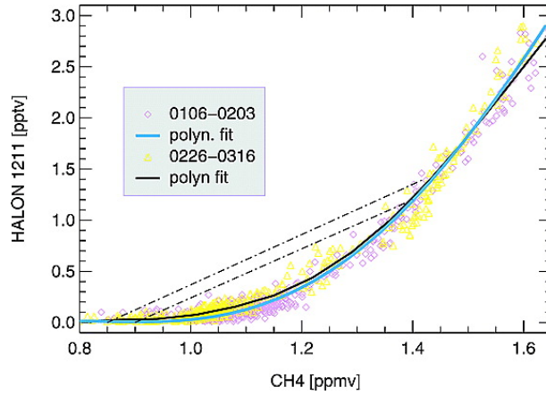
FIG. 4.3 – Corrélations entre CH_4 et Halon-1211 issues des vols ER-2 entre le 6 Janvier et le 16 Mars (Konopka et al., 2003 [129]). Les deux lignes pointillées représentent la zone où les lignes de mélange récents sont supposées être observées.
