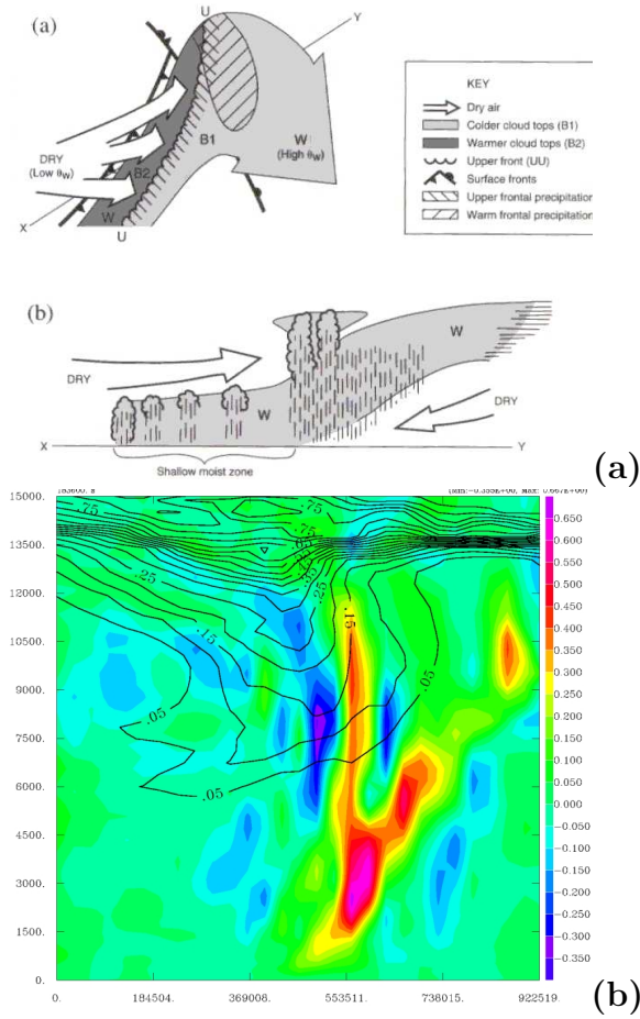
FIG. 2.16 – (a) Schéma du modèle conceptuel de split front (Browning and Monk, 1982). (b) Coupe verticale de vitesse verticale (m/s, en couleur) avec le pourcentage de traceur stratosphérique (iscontours noirs) valable le 16 Juillet à 21h.
