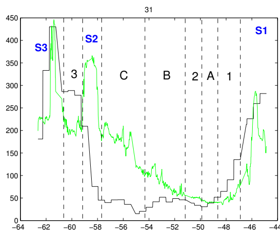
FIG. 2.6 – Ozone reconstruit RDF (ppbv, en noir) calculé à partir d’un run synthétique d’ozone flexpart en mode forward. La valeur d’ozone est calculée après 35h de rétro-trajectoire le long (a) du profil MOZAIC et (b) le long du vol croisière. L’ozone (ppbv) MOZAIC est représenté en vert sur ces 2 figures
