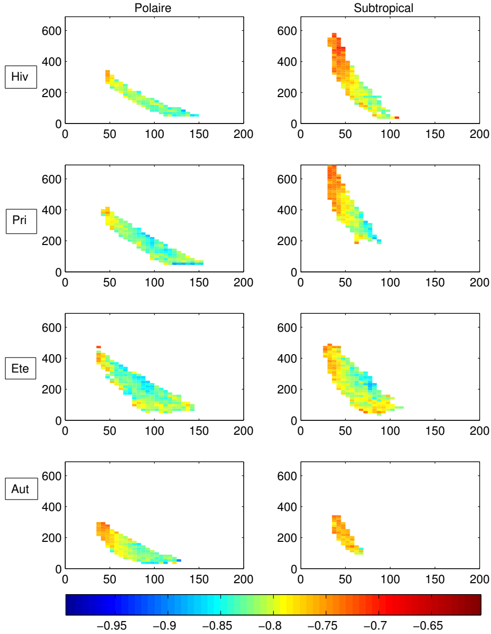
FIG. 4.12 – Diagrammes ozone/CO colorés par la corrélation temporelle moyenne après traitement de donnée. les quatres lignes correspondent aux quatres saisons. Les corrélations moyennes de la colonne de gauche sont obtenues pour des seuils en température potentielle traversant la tropopause polaire (seconde ligne du tableau 4.2). La colonne de droite correspond aux seuils en température potentielle traversant la tropopause subtropicale (première ligne du tableau 4.2).
