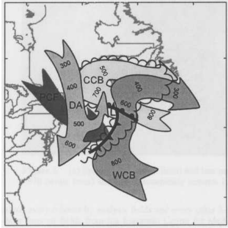
FIG. 1.2 – Schéma des flux isentropes dans une dépression à maturité aux moyennes latitudes, figurant la Cold Conveyor Belt (CCB), le Warm Conveyor Belt (WCB), et la Dry Intrusion (DA) avec les niveaux de pressions correspondants en hPa. Les fronts de surface chaud, froid et occlus sont représentés avec les symboles standards. Les nuages formés par les CCB et WCB sont aussi représentés. D'après Carlson, (1980) [35]; Bader et al., (1995) [19]; Cooper et al., (1998 [39], 2001 [41]).
