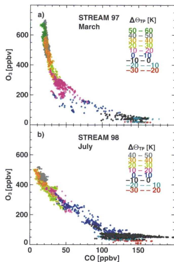
FIG. 4.4 – Graphique ozone/CO obtenu durant la campagne STREAM (Hoor et al., 2002 [81]). Les rapports de mélange d’ozone et CO sont donnés en ppbv. Le code de couleur indique la température potentielle. En haut pour la campagne de Mars, en bas pour la campagne de Juillet. Les pentes en Juillet sont de -4 à -6
