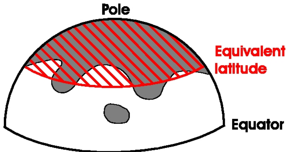
FIG. 4.18 – Schéma illustrant le concept de latitude équivalente (Hegglin et al., 2006 [83]). Une aire (couleur grise) entourée par un contour de PV sur une surface isentrope est transformée en un cercle dont l'air est identique, centré autour du pôle. La latitude de ce cercle est définie comme étant la latitude équivalente. Ainsi, une goutte froide avec un fort PV sur une surface isentrope donnée sera positionnée à une latitude plus haute.
