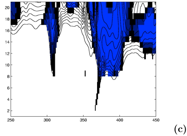
FIG. 4.20 – Isocontours de PV suivant une coupe zonale de 100^\circ en longitude, colorée par l'angle des surfaces PV sans filtrage FFT (en haut), avec filtrage FFT (milieu). L'image du bas représente la sélection en bleue des parties où la dérivée seconde des surface PV est positive.
