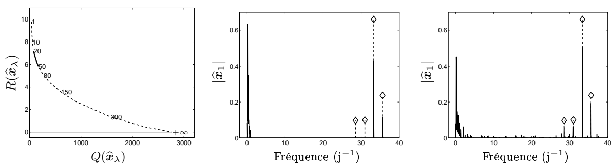
FIG. 5.5 – Sensibilité de l'estimation par pénalisation \ell^1 à la valeur du paramètre de régularisation. À gauche, courbe (Q(\hat{\mathbf{x}}_\lambda), R(\hat{\mathbf{x}}_\lambda)) paramétrée en \lambda . Le trait plein représente la zone fournissant une estimation acceptable. Au centre, sur-régularisation ( \lambda = 55 ) et à droite, sous-régularisation ( \lambda = 5 ). Les traits pleins représentent le module du spectre estimé et les \diamond les raies théoriques.
