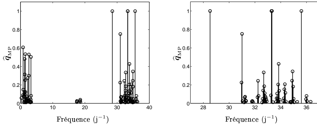
FIG. 5.27 – Données corrigées : moyenne estimée \hat{q}_{MP} pour la modélisation B-G_0 . À gauche, sur l'ensemble de la grille fréquentielle de P + 1 = 1001 points. À droite, entre 27 et 37 j^{-1} . Afin d'améliorer la lisibilité, seules les valeurs supérieures à 10^{-2} ont été représentées.
