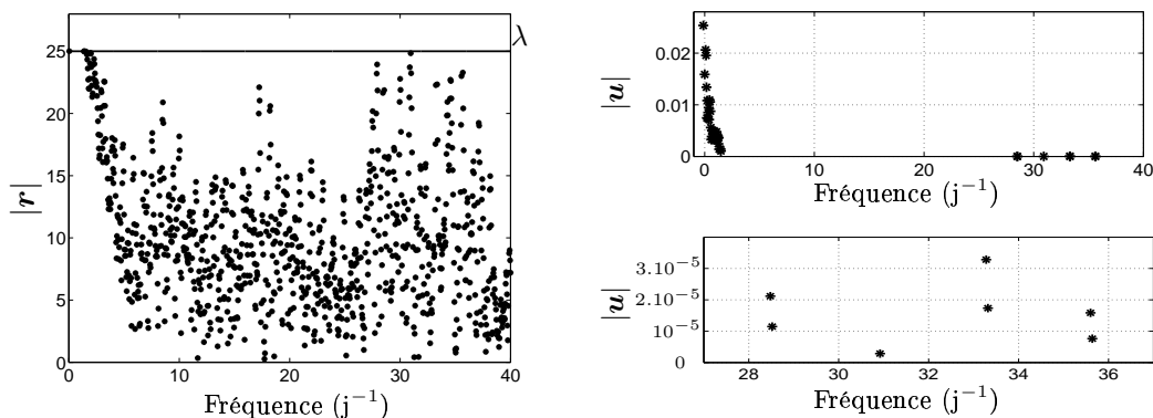
Test d'optimalité du minimiseur du critère J_1 en la solution \hat{x}_1 . À gauche, condition (i) : tracé de |r_k| pour les composantes nulles de x . Le trait plein représente le seuil de valeur \lambda . À droite, condition (ii) : valeurs en module de u_k = r_k + \lambda x_k / |x_k| pour les composantes non nulles de x .
