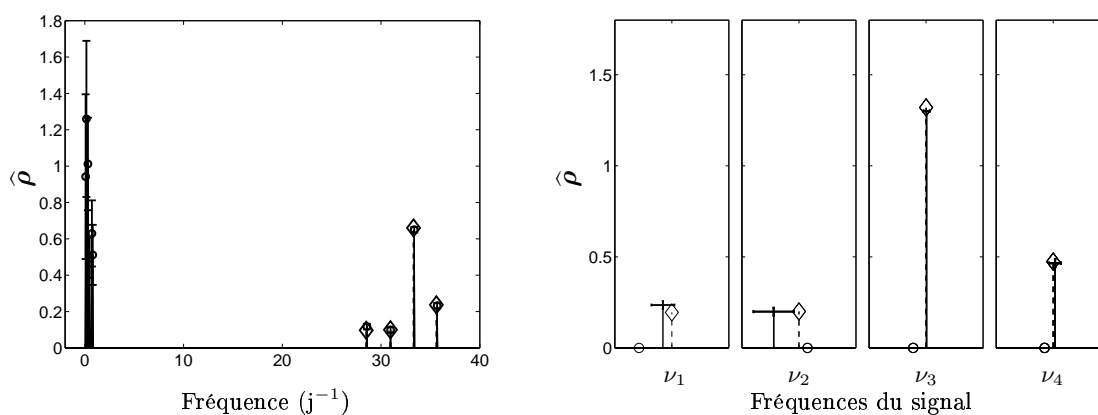
FIG. 5.13 – Estimation au sens du maximum a posteriori des amplitudes pour les fréquences localisées par \hat{q}_{MP} > 0.5 . À gauche, sur l'ensemble de la grille fréquentielle ; à droite, zoom en fréquence autour de chaque raie. Les barres d'erreur correspondent à \pm\sigma_k , où \sigma_k est l'écart-type associé, et les \diamond représentent les raies théoriques. Chaque fenêtre en fréquence sur la figure de droite couvre une plage de la même largeur qu'à la figure 5.10, soit 8 \times 10^{-2} j^{-1} .
