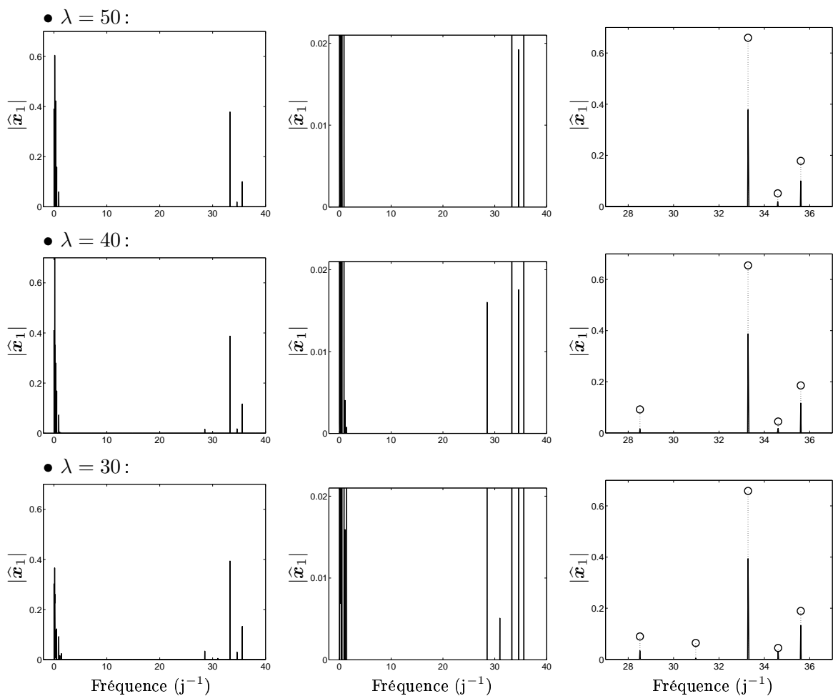
FIG. 5.15 – Résultats d'estimation par minimisation d'un critère pénalisé pour \lambda = 50 à \lambda = 30 . À gauche, estimé en module sur l'ensemble de la grille fréquentielle de P + 1 = 5001 points. Au centre, zoom en amplitude pour les faibles valeurs. À droite, zoom en fréquence sur l'intervalle \mathcal{I} = [27 j^{-1}, 37 j^{-1}] . Les traits pleins représentent le module du spectre estimé et les \circ correspondent à la réestimation a posteriori par moindres carrés régularisés des amplitudes localisées par les pics de |\hat{\mathbf{x}}_1| .
