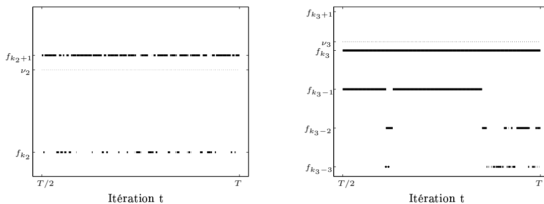
FIG. 5.9 – Échantillons de Bernoulli q_{k_j}^{(t)} au fil des itérations. À gauche, pour les fréquences autour de \nu_2 ; à droite, pour les fréquences autour de \nu_3 . Le trait plein marque les valeurs q_{k_j}^{(t)} = 1 .
