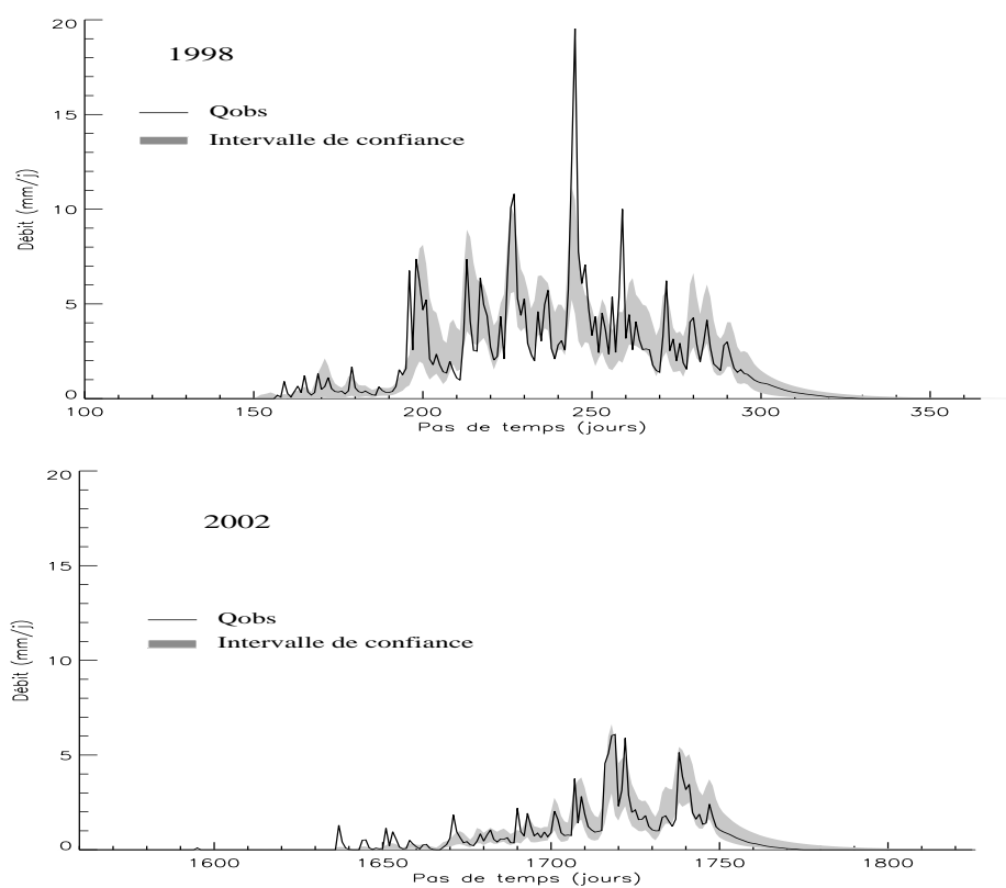
FIG. 5.23: Intervalles prédictifs (interquantile 90%) sur les débits simulés par TOPAMMA. Exemples de 1998 et 2002
