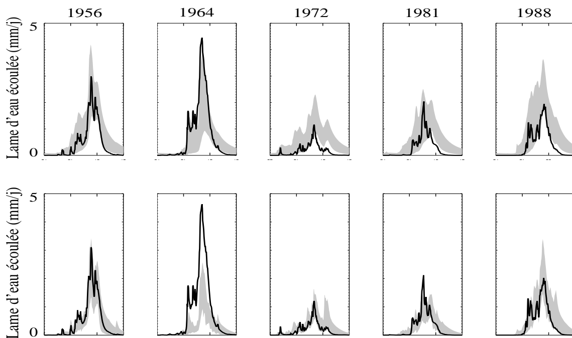
FIG. 6.5: Exemples d'hydrogrammes observés et intervalles de confiance à 90% sur les simulations, pour GR4J (en haut) et TOPAMMA (en bas)
