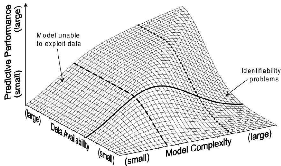
FIG. 2.4: Schématisation de la relation entre complexité du modèle, données disponibles et performances du modèle (d'après Grayson et Blöschl 2000)
