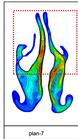
Figure 3 - 18 : Sections transversales des cavités nasales du modèle plastiné représentant les contours de vitesses normalisées par la vitesse moyenne sur chaque section. Les différentes sections sont localisées à l'entrée des narines (plan-1), juste après la région de la valve nasale (plan-3), avant l'apparition des cornets (plan-5), au niveau de la tête des cornets (plan-6), dans la région des cornets (plan-7) et enfin vers la queue des cornets (plan-14) un peu avant la région du nasopharynx. La position de ces sections est visible sur la Figure 3-1(a). Le débit inspiratoire simulé dans les deux cas est Q_{exp} = 216 ml/s.
