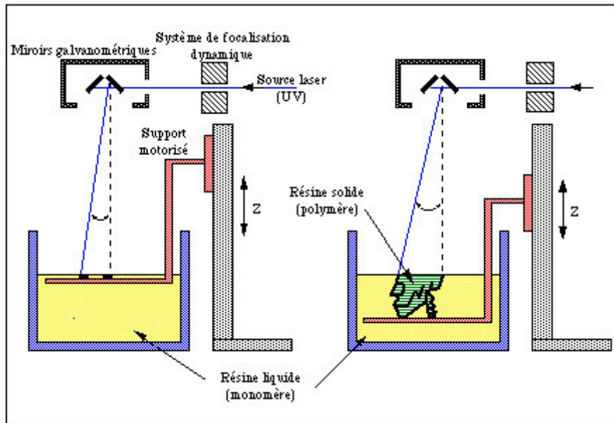
Figure 2-6: Schéma représentant le principe de stéréolithographie ( http://www.valla.fr/nlds/modules/upload/upload/sla%20principe.jpg )
