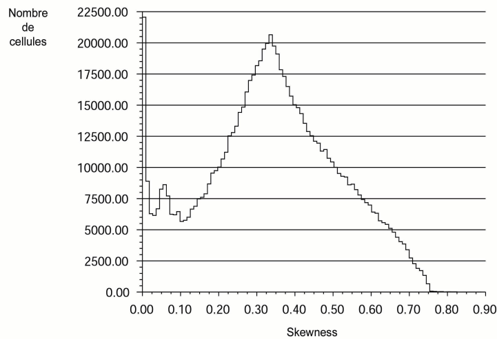
Figure 2-21 : Qualité du maillage volumique du modèle du nez plastiné réalisé par la société Fluent avec le logiciel TGrid ® . Graphique représentant le nombre d'élément pour chaque valeur de « skewness » en fonction des valeurs du « skewness ». La valeur maximale du « skewness » pour ce maillage volumique est de 0,812.
