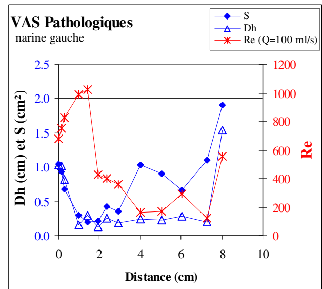
Figure 3 -6 : Figures représentant, pour chaque narine (droite ou gauche) de chaque modèle géométrique, l'évolution de l'aire ( S ), du diamètre hydraulique ( D_h ) et du nombre de Reynolds ( Re ) le long de l'axe de chaque cavité.
