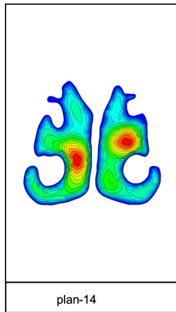
Figure 3 - 18 : Sections transversales des cavités nasales du modèle plastiné représentant les contours de vitesses normalisées par la vitesse moyenne sur chaque section. Les différentes sections sont localisées à l'entrée des narines (plan-1), juste après la région de la valve nasale (plan-3), avant l'apparition des cornets (plan-5), au niveau de la tête des cornets (plan-6), dans la région des cornets (plan-7) et enfin vers la queue des cornets (plan-14) un peu avant la région du nasopharynx. La position de ces sections est visible sur la Figure 3-1(a). Le débit inspiratoire simulé dans les deux cas est Q_{exp} = 216 ml/s.
