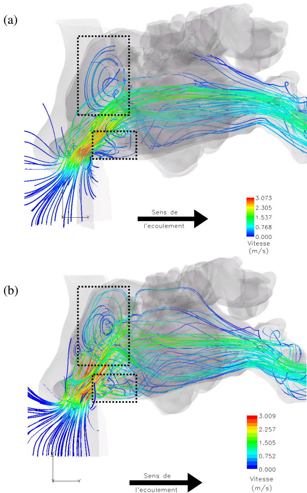
Figure 3 - 14 : Visualisation des lignes de courant en 3D pour les simulations effectuées sur la base d'un débit inspiratoire Q_{exp} = 216 \text{ ml/s} (a) dans notre laboratoire et (b) par la société Fluent. Les deux simulations ont été effectuées avec un modèle d'écoulement laminaire. Les lignes de courant sont colorées en fonction de l'amplitude de la vitesse. Les zones encadrées en pointillés sont des régions de fortes recirculations pour l'écoulement.
