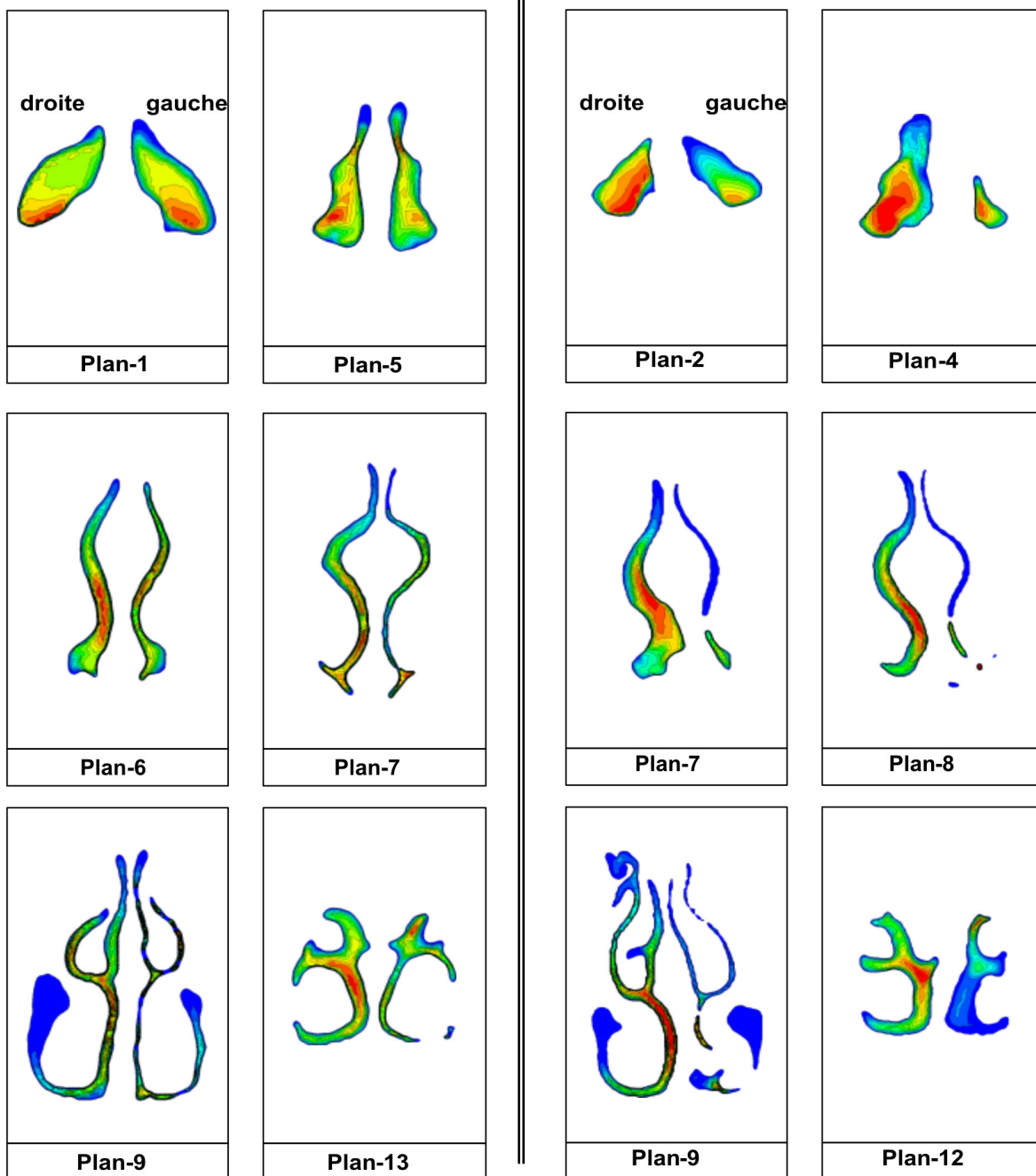
Figure 3 - 22 : Contours de vitesses normalisées sur quelques sections transversales des cavités nasales des modèles de VAS saines (A) et pathologiques (B). Les différentes sections sont localisées à l'entrée des narines (plan-1 pour le modèle de VAS saines vs plan-2 pour le modèle de VAS pathologiques), avant l'apparition des cornets (plan-5 vs plan-4), au niveau de la tête des cornets (plan-6 vs plan-7), dans la région des cornets (plan-9 vs plan 9) et enfin vers la queue des cornets (plan-13 vs plan-12) un peu avant la région du nasopharynx. La localisation des différentes sections transversales de ces deux modèles de VAS est visible sur les Figures 3-1(b) et (c). L'orientation droite/gauche est notée pour la première section de chaque modèle et reste valable pour les autres sections.
