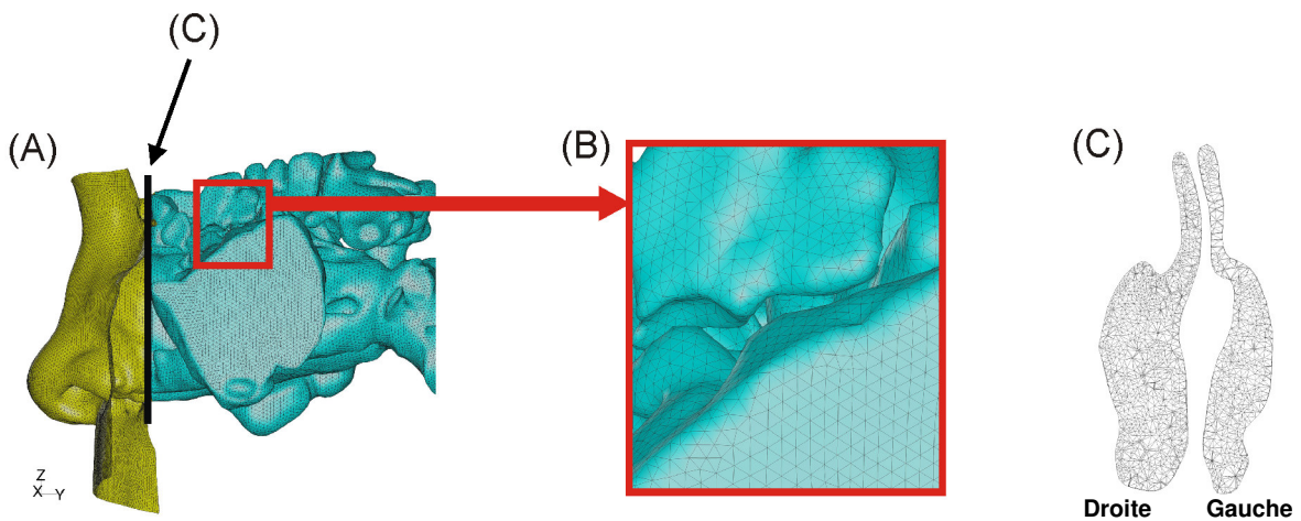
Figure 2-22 : (A) Visualisation de l'enveloppe surfacique d'une partie du maillage volumique du modèle de nez plastiné réalisé avec le logiciel TGrid ® . (B) Vue détaillée du maillage surfacique. Les deux couleurs différentes utilisées pour la représentation graphique du maillage surfacique permettent juste de visualiser une partie du découpage de la géométrie qui a été nécessaire lors du processus de maillage. (C) Vue détaillée du maillage sur une section transversale des cavités nasales.
