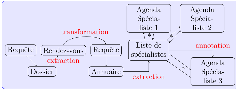
FIG. 1.2 – Les documents échangés entre l’agent de Lucie et les services Internet des autres acteurs. Les échanges de documents XML sont enchaînés avec des extractions, transformations ou annotations de documents. (Les parties avec * ne sont pas détaillées).
