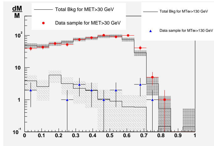
FIG. 5.26 – Distribution en \frac{dM}{M} pour MLQ = 200 GeV. Les données apparaissent sous forme de points et de triangles, en histogramme noir le bruit de fond total.
