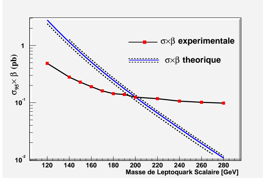
FIG. 5.17 – limite à 95% de degré de confiance sur la section efficace fois le rapport de branchement en fonction de la masse du leptoquark scalaire (sous forme de carrés). Les sections efficaces théoriques calculées au second ordre y sont présentées pour différents facteurs de normalisation : M_{LQ} (line pleine), M_{LQ}/2 et M_{LQ} * 2 (lignes hachurées).
