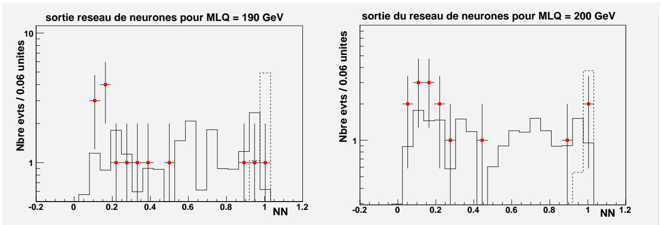
FIG. 5.28 – Distributions de la réponse des réseaux de neurones pour les masses de leptoquark de 190 GeV (à gauche) et de 200 GeV (à droite). Les données apparaissent sous forme de points, en trait noir le bruit de fond total estimé. En pointillés apparaît le signal attendu pour un rapport de branchement de 0.5.
