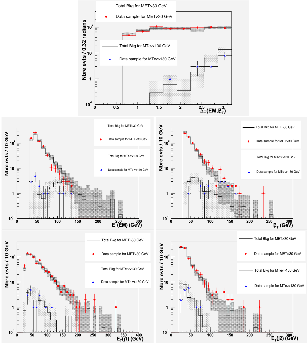
FIG. 5.13 – Les données apparaissent sous forme de points, en trait noir le bruit de fond total. Pour E_T > 30 \text{ GeV} , apparaissent successivement les distributions de \Delta\phi(EM, \vec{E}_T) , l'énergie transverse de l'électron, l'énergie manquante, et les énergies transverse des deux premiers jets. Pour chacune des figures, deux histogrammes apparaissent, l'un avec la coupure en M_T(ev) > 130 \text{ GeV} et l'autre sans.
