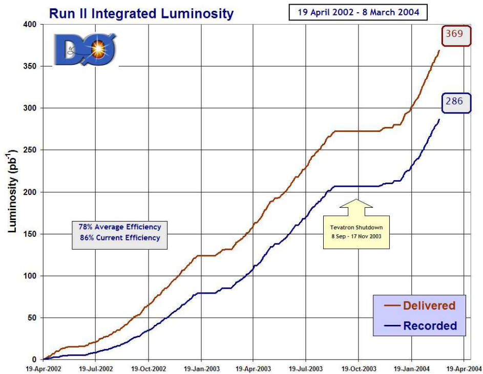
FIG. 2.14 – Evolution de la luminosité intégrée délivrée par le Tevatron et celle enregistrée par l'expérience D\emptyset . la courbe représentant la luminosité délivrée est au-dessus de celle représentant la luminosité enregistrée.
