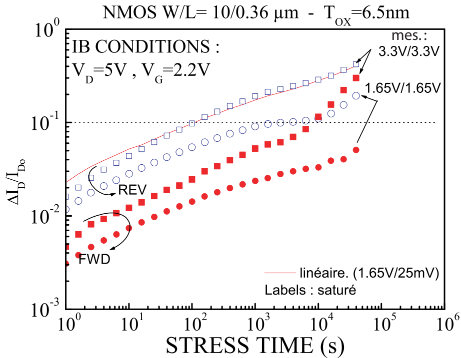
FIG. III.26 – Variation de la dégradation relative du courant de Drain au court d'un stress au maximum du courant substrat ( V_{DS} = 5V ) pour un transistor NMOS de la technologie T2.
