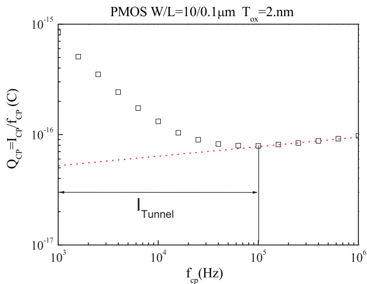
FIG. II.23 – Décrochage typique dû à une forte composante tunnel dans un mesure CP (Signal sinusoïdal, amplitude \Delta V_A = 2.4\text{V} ) [20].
