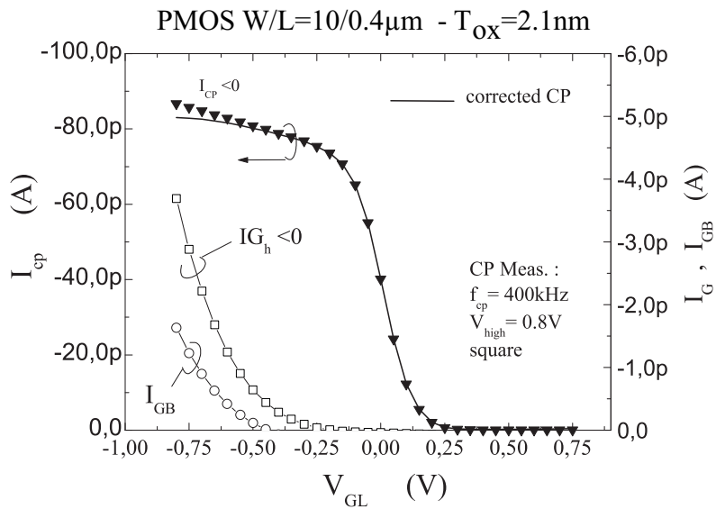
FIG. II.22 – Comparaison des courbes CP – V_{GL} avec les courbes de courant de Grille ( I_G ) et le courant tunnel ( I_{GB} ) calculé avec (II.47).
