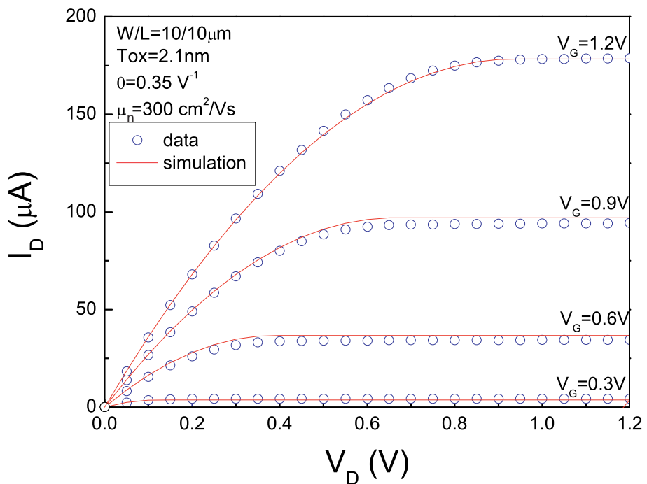
FIG. I.24 – Modélisation du courant de Drain suivant V_{DS} en régime saturé avec réduction de mobilité à un coefficient pour un canal N long ( W/L = 10/10\mu\text{m} ) et oxyde ultra mince T_{ox} = 2.1\text{nm} .
