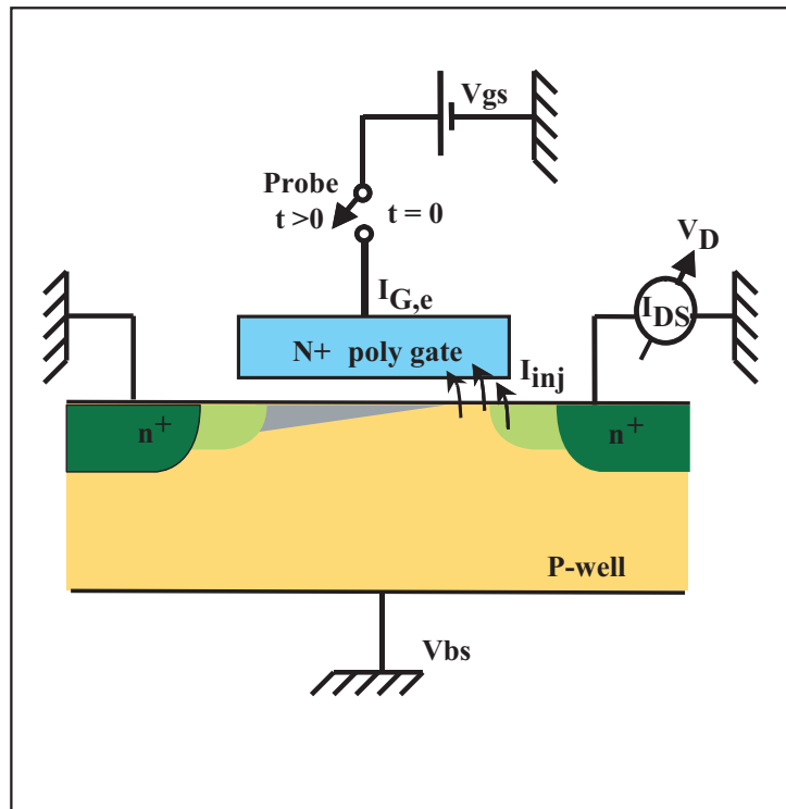
FIG. II.27 – Principe de la mesure par Grille Flottante.
