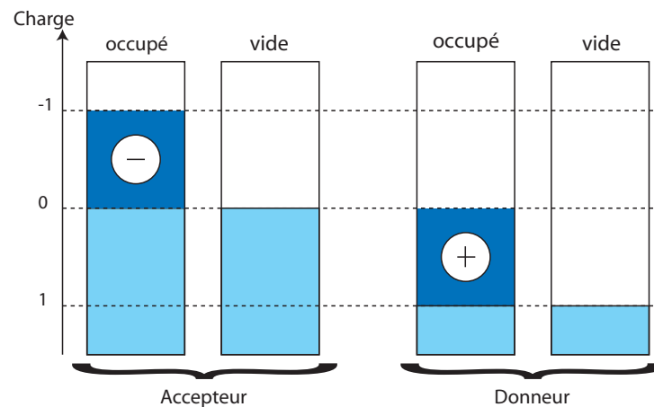
FIG. I.6 – représentation des pièges suivant leur type vis à vis des électrons.
