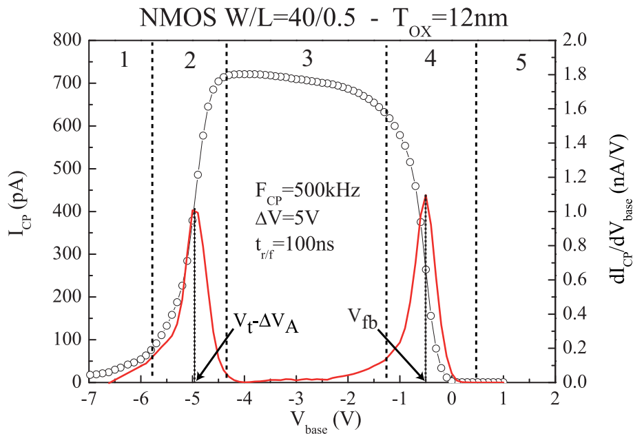
FIG. II.16 – Mesures de pompage de charges à amplitude constante sur transistor NMOS W/L = 40/0.5\mu m , T_{ox} = 12nm , les fronts du signal ont une durée de 100ns, le rapport cyclique est de 50%.
