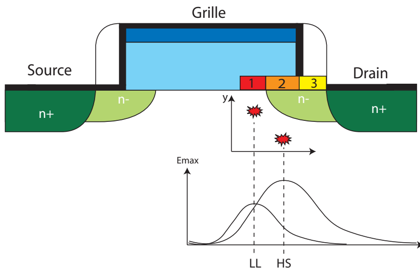
FIG. III.58 – Localisation des pics de champ les transistors PMOS des technologies T3 et T4.
