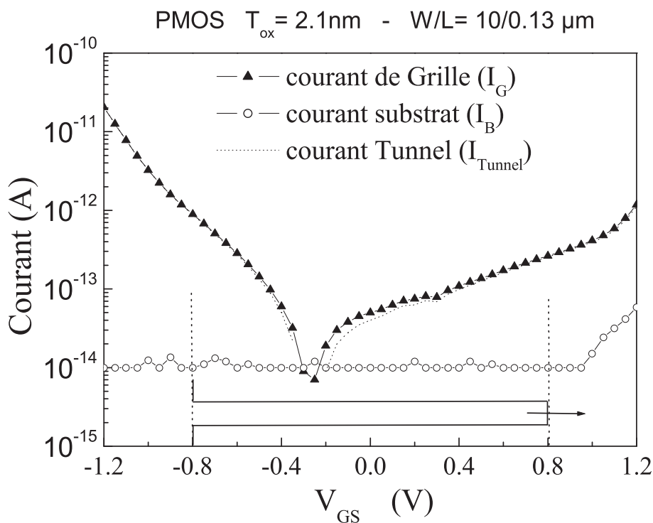
FIG. II.21 – Courant de Grille et de substrat nécessaires au calcul de I_{GB} = I_G - I_B
