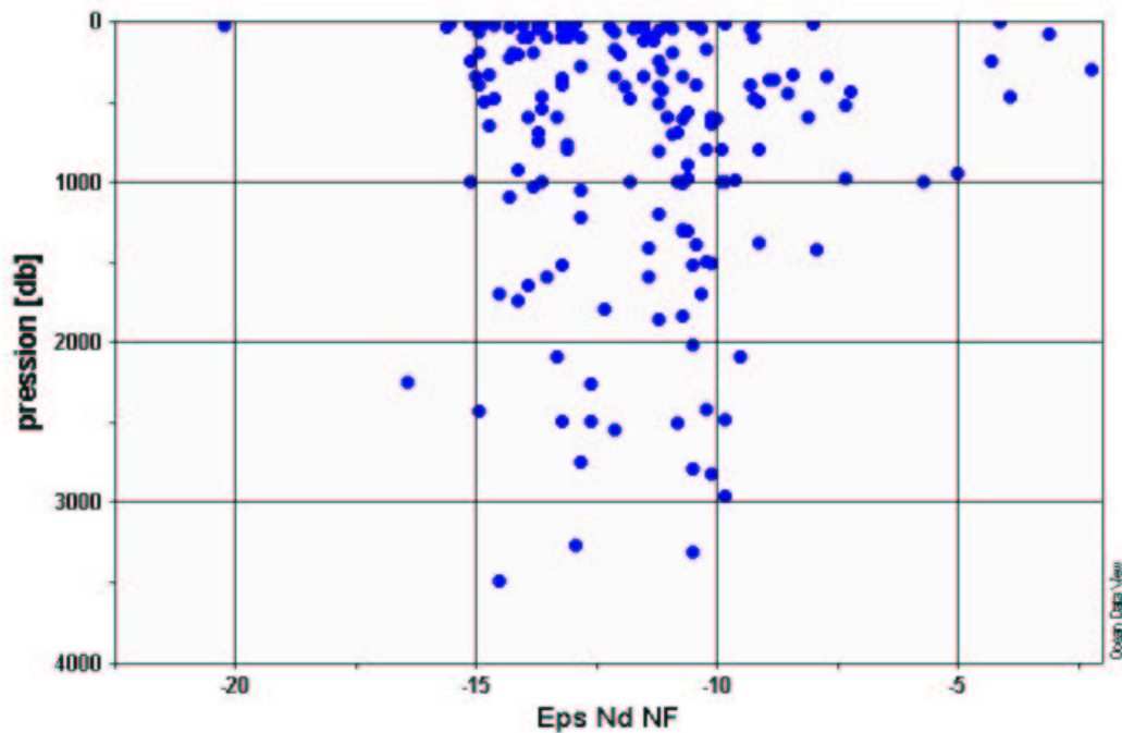
FIG. 4.6 –: Ensemble des C.I. de Nd de la campagne Signature/GINS en fonction de la profondeur. Le nombre de données inférieures ou égales à -15.0 est très faible. Ces dernières correspondent à des échantillons prélevés dans le bassin du Labrador (outre ceux de la station 12).
