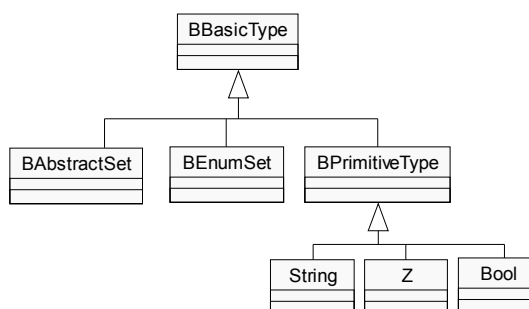
FIG. 3.9 – Spécialisations de BBasicType
