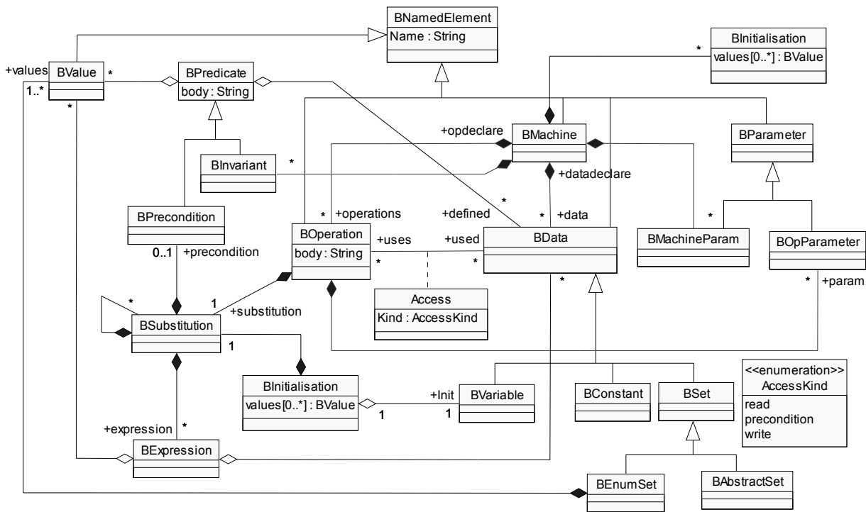
FIG. 3.6 – Méta-modèle UML pour la spécification de machines abstraites B
