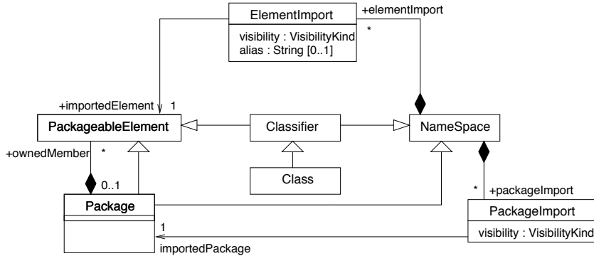
FIG. 5.1 – Extrait du méta-modèle UML relatif aux dépendances entre paquets
