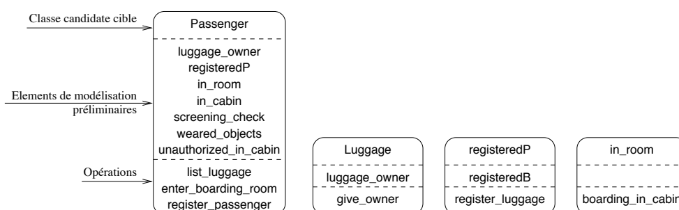
FIG. 7.8 – Modèle de contextes issu de la fusion de SecureFlightBoarding et SecureFlightRegistration
