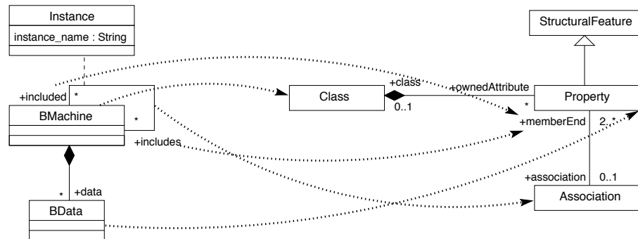
FIG. 5.4 – Schéma de transformation « Inclusion entre machines – Cas 2 »
