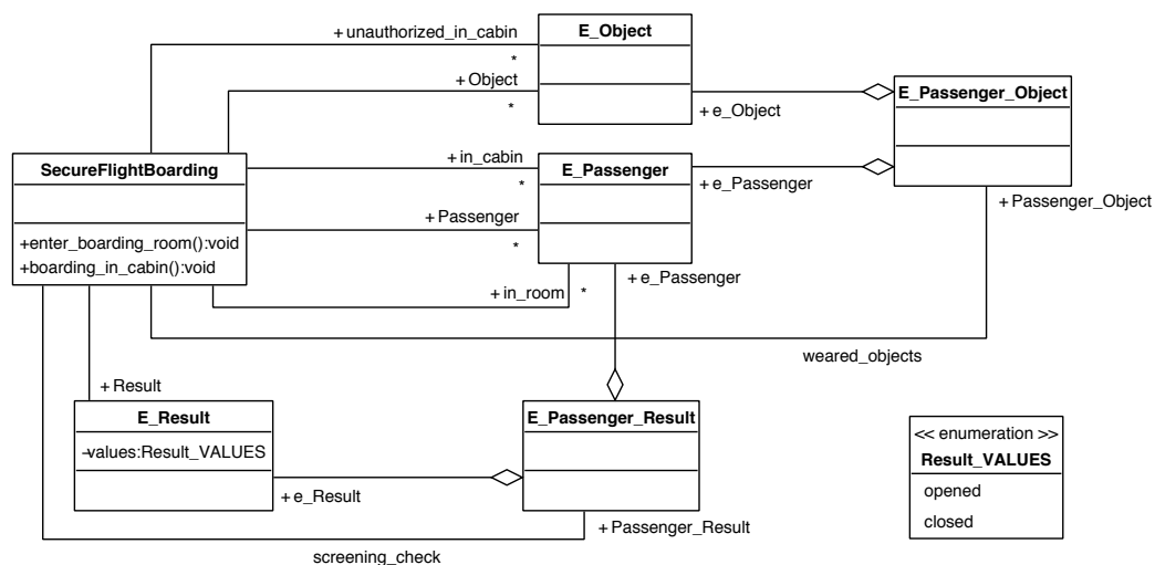
FIG. 5.14 – Application de l'approche de (Voisinet, 2004, Tatibouet et al. , 2002) sur la machine SecureFlightBoarding
