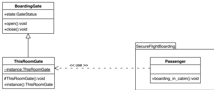
FIG. 5.8 – Application du patron « Singleton »
