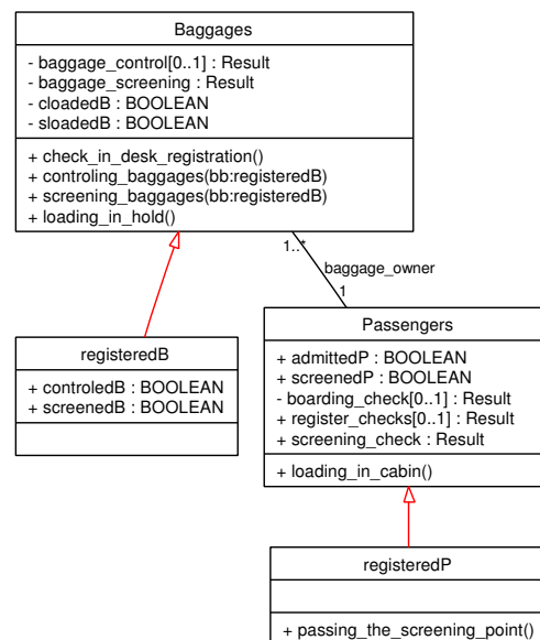
FIG. 9.12 – Diagramme de classes issu de l'un des modèles de contextes dont la pertinence moyenne est égale à 95%
