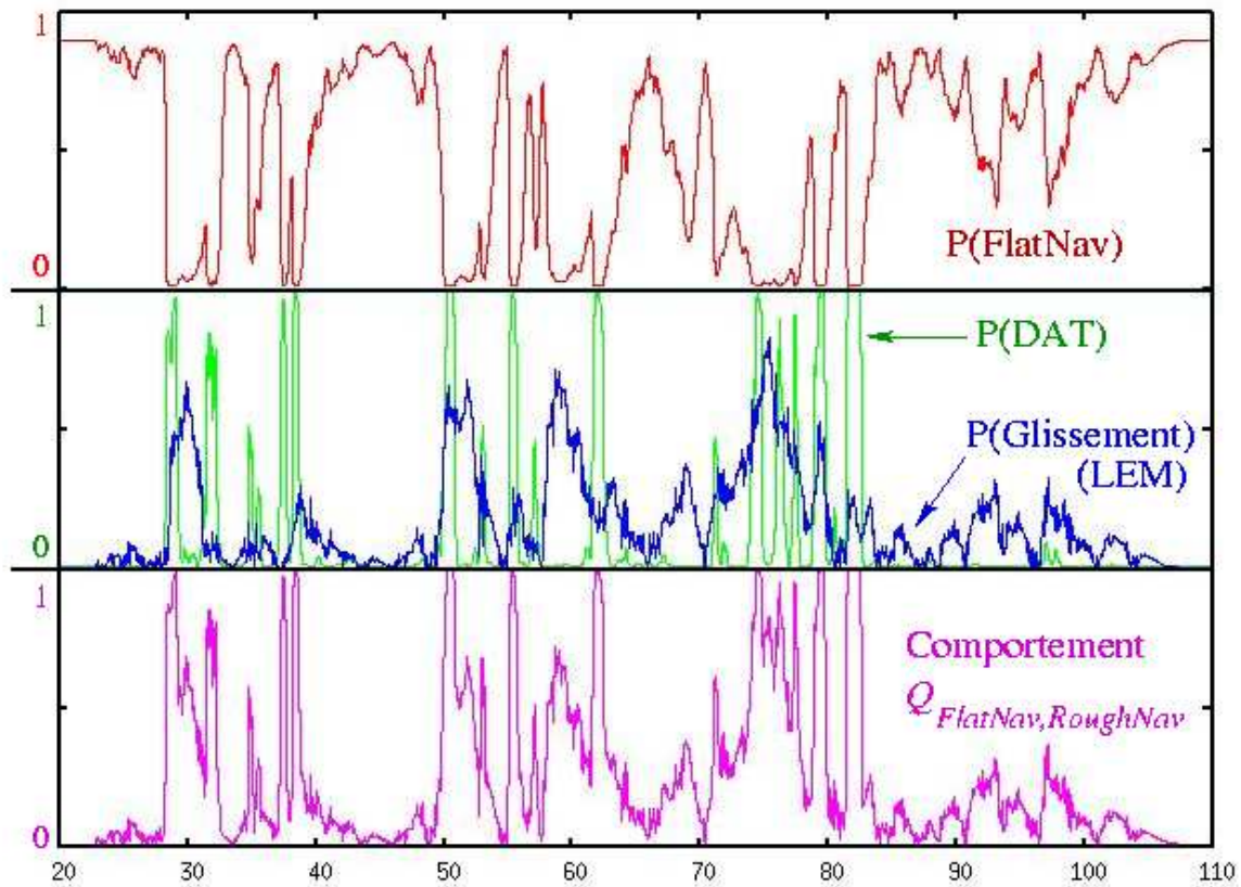
FIG. 6.10 – Un autre exemple dans la même situation que la figure précédente mais avec des probabilités d’observation du contexte différentes (toujours fixées par un opérateur humain) : p(O|Plat) = p(O|FlatNav) = 0.60 , p(O|Accidente) = p(O|RoughNav) = 0.38 et p(O|Obstacle) = p(O|Stop) = 0.02 . Les probabilités initiales sont quant à elles : P(FlatNav) = 0.8 , P(RoughNav) = 0.19 et P(Stop) = 0.01 .
