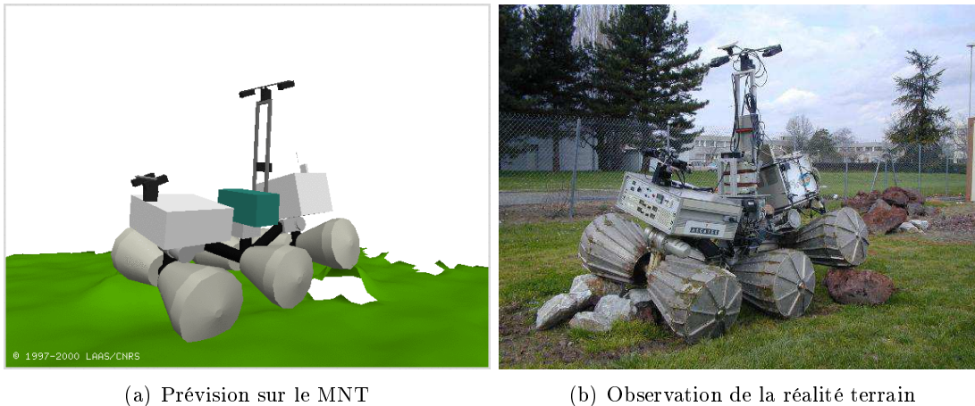
FIG. 3.12 – Illustration du posé de robot sur un terrain accidenté : comparaison entre prédiction sur le MNT et observation.
