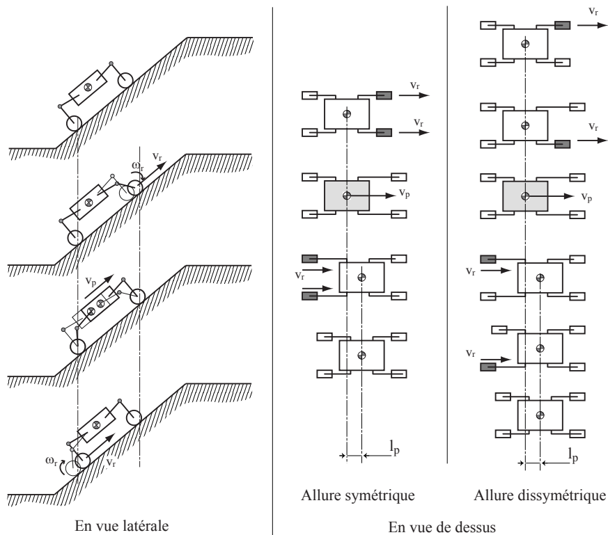
FIG. B.2 – Illustration du mode de locomotion péristaltique pour un robot hybride roue-patte comme Hylos, d’après [Grand, 2004].
