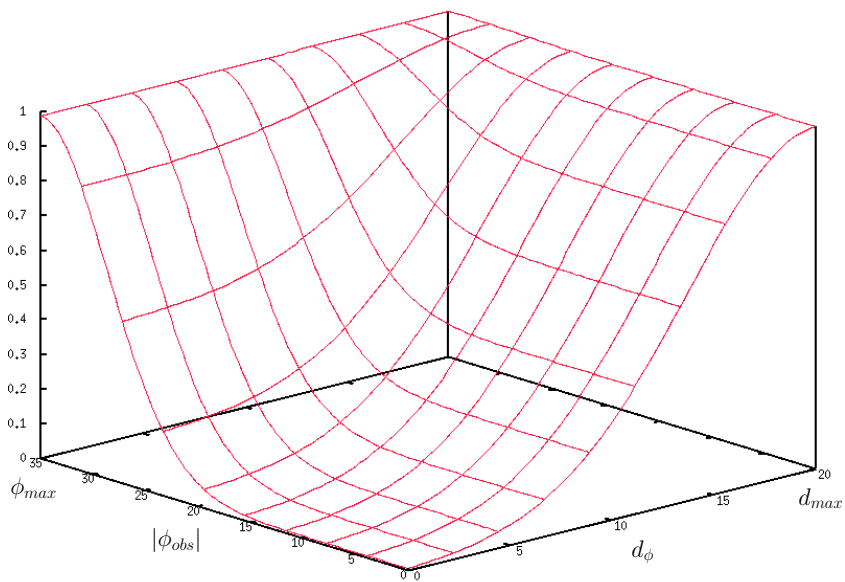
FIG. 5.11 – Pseudo-probabilité de comportement avec l'influence de la limite angulaire \phi_{max} .
