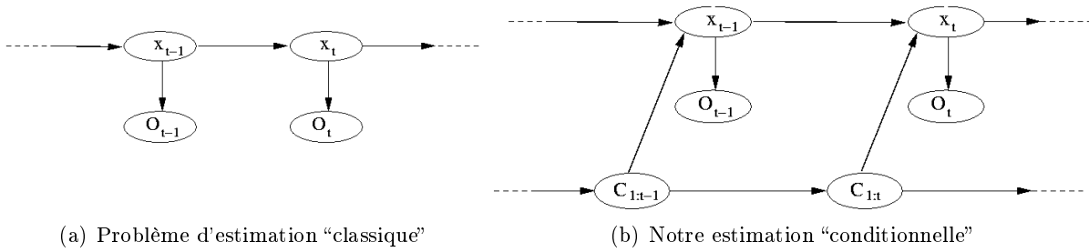
FIG. 2.6 – Graphe de dépendance orienté de la chaîne de Markov cachée des variables x_{0:t} , O_{1:t} (et C_{1:t} ).
