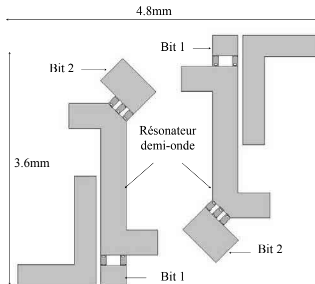
Figure III - 35: Topologie du filtre digital.
