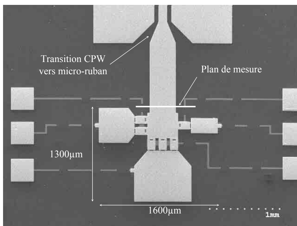
Figure III - 13: Capacité digitale avec sa transition CPW vers micro-ruban.
