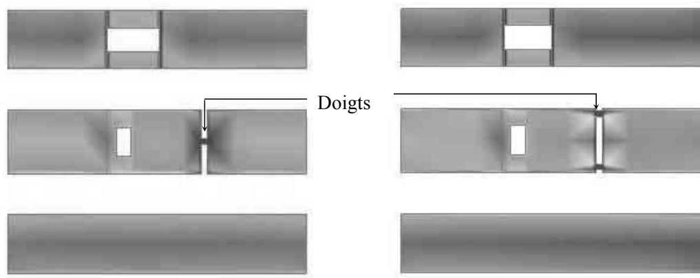
Figure II - 48: Distribution des courants pour un commutateur à 1 et 2 doigt(s) de contact.
