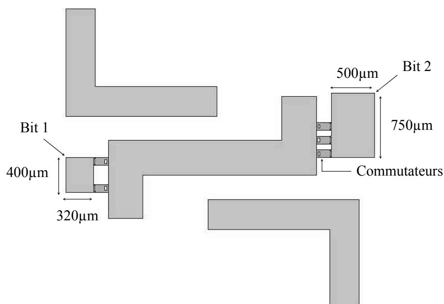
Figure III - 33: Charges capacitatives implémentées sur le résonateur.
