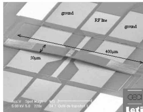
Figure I - 24: Commutateur à contact ohmique développé par le LETI, ST Microelectronics et L'IRCOM.
