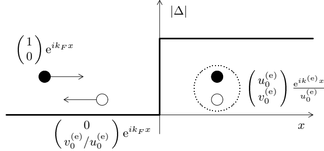
Fig. 5.1. Andreev reflection
