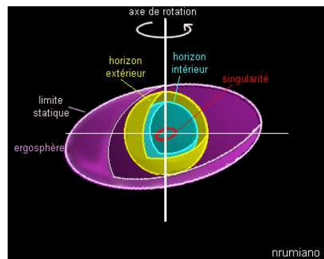
FIG. C.3 – Illustrations d'un trou noir de Kerr.
