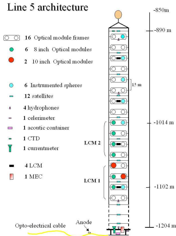
FIG. 2.27 – Schéma de la ligne 5, le démonstrateur d'ANTARES.
