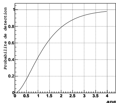
FIG. 6.18 – Probabilité de détection en fonction du temps, pour des cannonballs moyens dans le modèle de volume, si la distribution des angles de vue est uniforme (figure 6.15).
