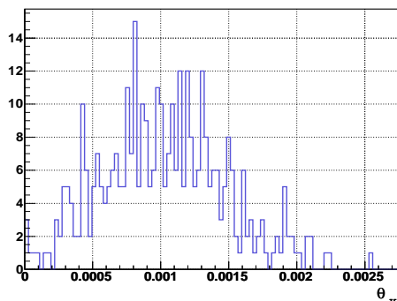
FIG. 6.13 – Distribution des angles de vue tirés aléatoirement sur une fonction de Gauss, centrée en \theta_v = 10^{-3} et de largeur 5 \times 10^{-4} . Le nombre d'événements associé est utilisé pour la figure 6.14.
