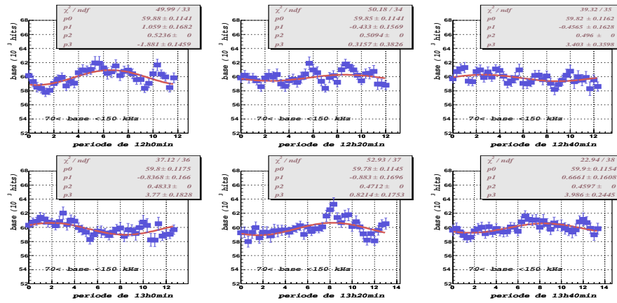
FIG. E.15 – Lignes de base repliées sur 12 h à 13h40. ( 70 < \text{base} < 150 kHz).
