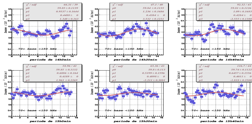
FIG. E.16 – Lignes de base repliées sur 14 h à 15h40. ( 70 < \text{base} < 150 kHz).
