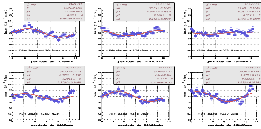
FIG. E.14 – Lignes de base repliées sur 10 h à 11h40. ( 70 < \text{base} < 150 kHz).
