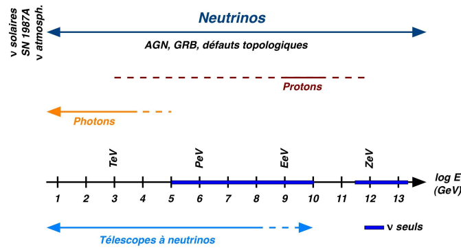
FIG. 1.5 – Domaine d'énergie couvert par les différents messagers. Les neutrinos sont présents sur tout le spectre et sont les seuls entre 10^5 et 10^{10} GeV ainsi qu'au-delà de 10^{12} GeV.
