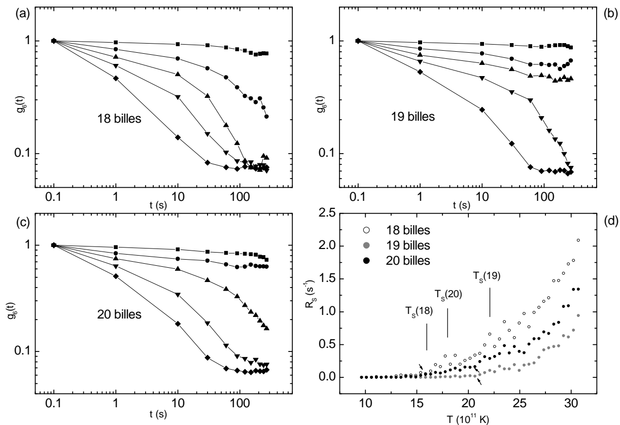
FIG. 9.2 : (a-c) : Variation des fonctions de corrélation orientationnelle g_6 en fonction du temps (échelle log-log) pour 5 températures : (■) T = 9.6 \times 10^{11} K , (●) T = 13.0 \times 10^{11} K , (▲) T = 17.8 \times 10^{11} K , (▼) T = 23.0 \times 10^{11} K , (◆) T = 30.2 \times 10^{11} K ; (a) N = 18 , (b) N = 19 et (c) N = 20 . (d) : Taux de sauts R_S dans les trois systèmes en fonction de la température. Les flèches indiquent la température à laquelle le deuxième état excité a été observé pour la première fois. Les températures seuil T_S(N) sont définies dans le texte.
