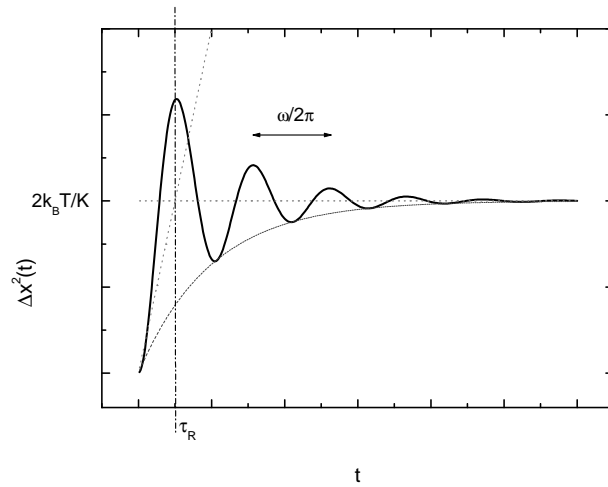
FIG. B.1 : Comportement général du déplacement quadratique moyen \Delta x^2(t) dans un puits harmonique, pour un amortissement faible.
