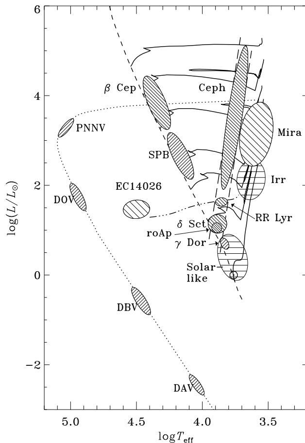
FIG. 1.6 – Diagramme HR (Hertzsprung-Russell) schématisant la position de différentes classes d'étoiles pulsantes (diagramme tiré de Christensen-Dalsgaard 2003).
