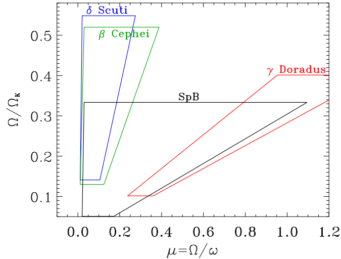
FIG. 1.15 – Domaines occupés par différentes classes d'étoiles dans un diagramme \Omega/\Omega_K - \mu , où (\Omega/\Omega_K)^2 correspond au rapport entre la force centrifuge et la gravitation et \mu au rapport entre l'échelle de temps associée aux pulsations et celle associée à la force de Coriolis (diagramme adapté de Goupil & Talon 2002).
