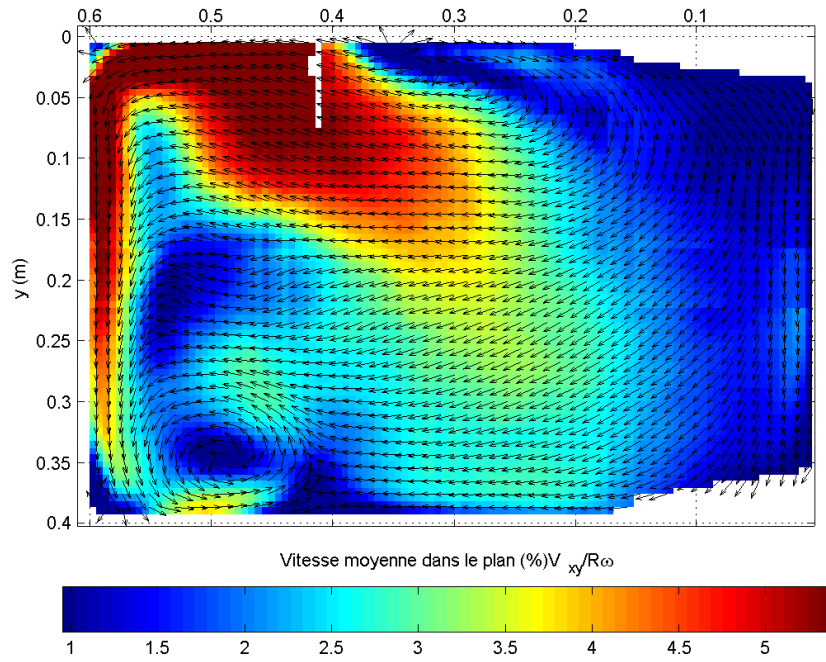
FIG. 7.2 – Plan G : Simulation k - \epsilon réalisable
