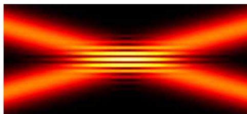
FIG. 5.1 – Franges d'interférence
