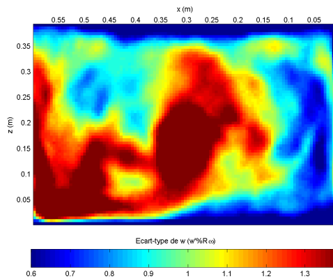
FIG. 7.36 – Plan E : \overline{w'^2} (LES Kim)
