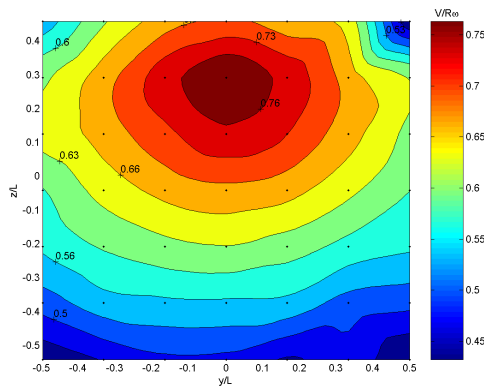
FIG. 5.18 – Vitesse moyenne
