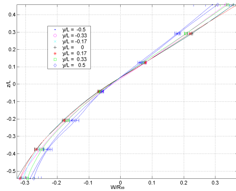
FIG. 5.27 – Vitesse verticale
