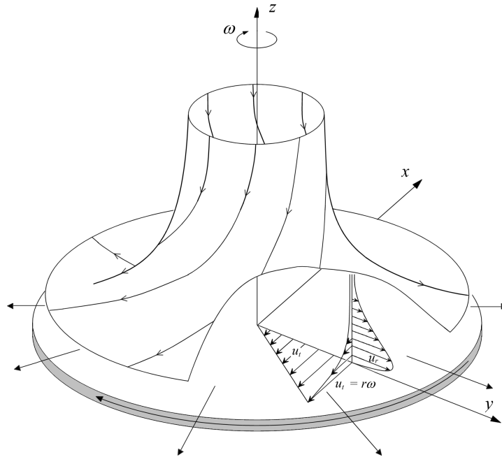
FIG. 2.1 – Ecoulement laminaire au voisinage d'un disque en rotation
