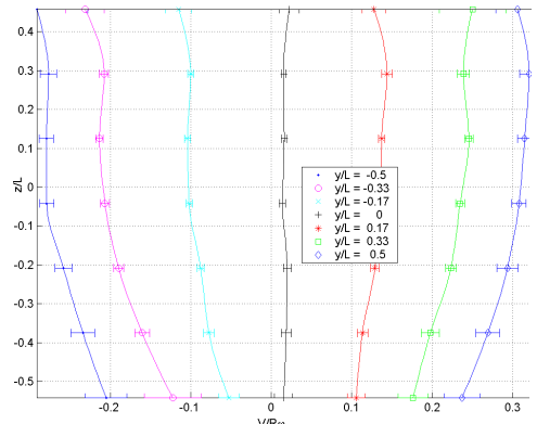
FIG. 5.26 – Vitesse horizontale
