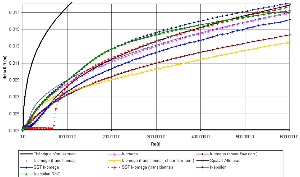
FIG. 2.8 – Epaisseur \delta_{0.9} de la couche limite
