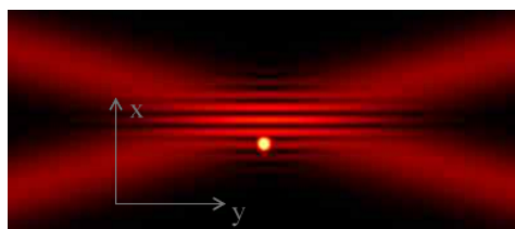
FIG. 5.2 – Transit d'une particule
