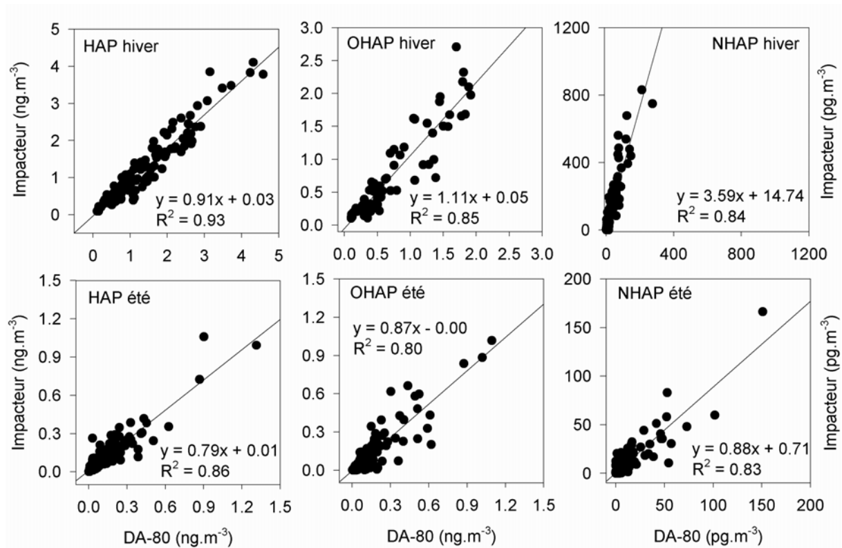
Figure IV.2 : Comparaison des concentrations particulières des HAP, OHAP et NHAP déterminées par la méthode classique de filtration (DA-80, tête PM 10 ) et par un impacteur en cascade en période hivernale et estivale (tous les sites de prélèvements confondus).
