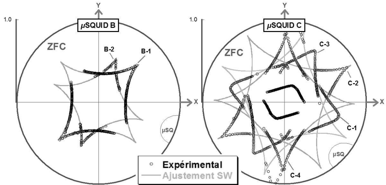
FIG. 4.27 – Champs de retournement d'agrégats de cobalt posés sur CoO après une procédure ZFC. L'ajustement des astroïdes est réalisé avec le modèle de Meiklejohn et Bean appliqué à des agrégats individuels.
