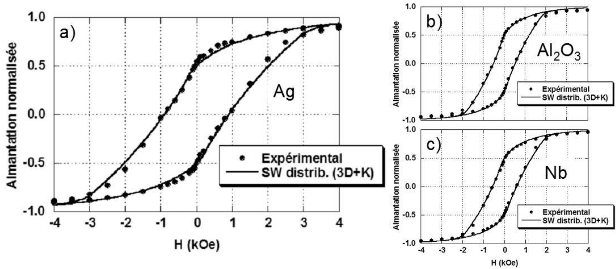
FIG. 3.6 – a) Aimantation d'une multicouche d'agrégats de cobalt dans l'argent (type 1 ); b) Aimantation d'agrégats de cobalt recouverts d'alumine (type 2 (a) ); c) Aimantation d'agrégats de cobalt recouverts de niobium (type 2 (b) ). Les courbes en trait plein correspondent au meilleur ajustement obtenu avec le modèle de Stoner-Wohlfarth tenant compte d'une distribution 3D des axes d'anisotropie et d'une distribution homogène des constantes d'anisotropie entre K_{min} et K_{max} . Les aimantations sont normalisées par rapport à l'aimantation totale des agrégats.
