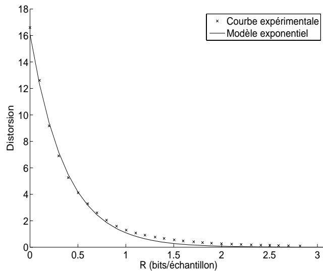
FIG. 4.1: Comparaison des courbes de distorsion en fonction du débit obtenues expérimentalement et à partir du modèle exponentiel (construit à partir de 3 points de débit 0,2; 0,4 et 0,6 bits par échantillon) - sous-bande D3 de l'image Lena.
