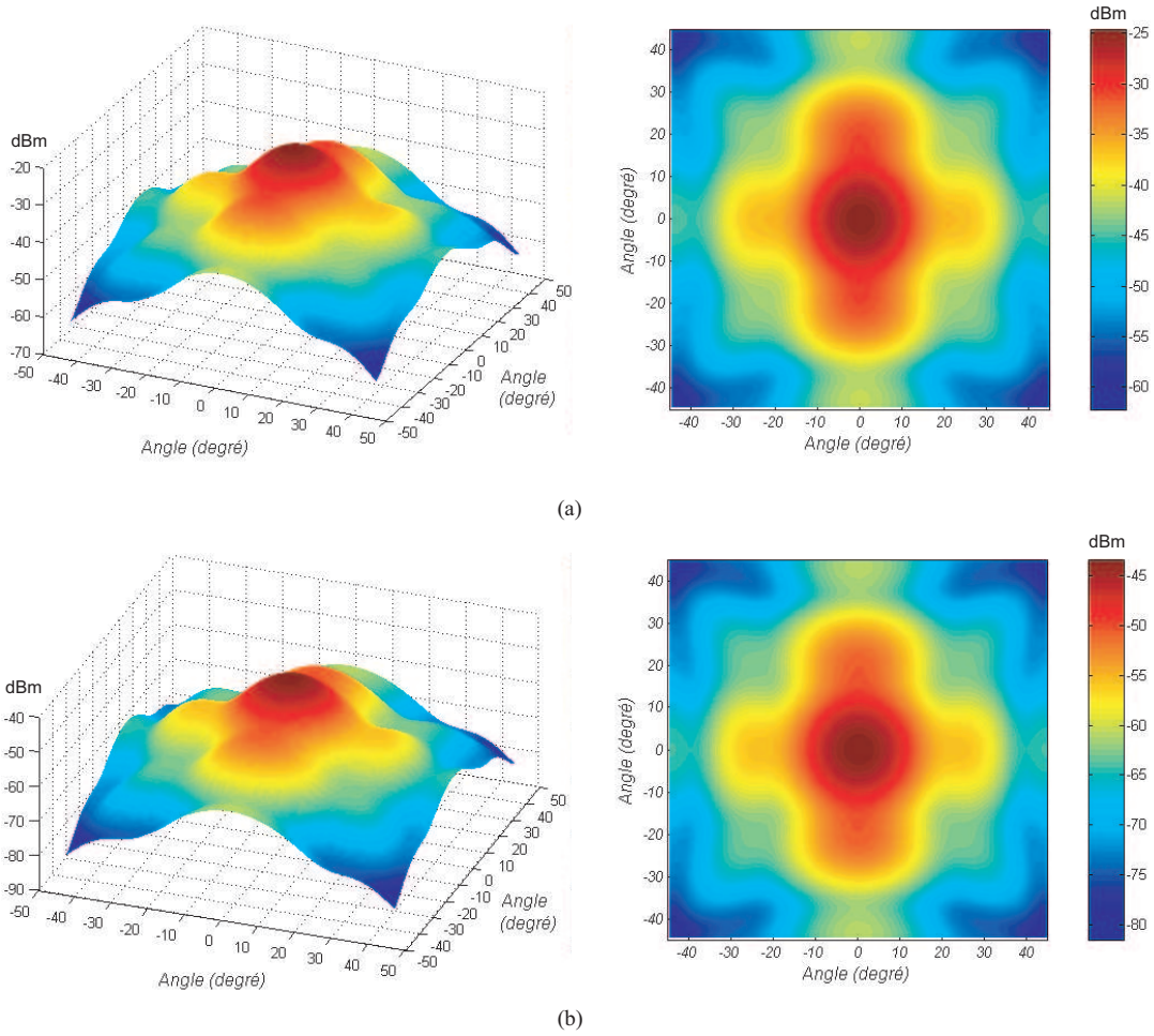
Fig. 5.13: Distribution de puissance de rayonnement ( P=1 dBm) de l'antenne cornet pyramidal à 60 GHz sur un surface plane éloignée de l'antenne de (a) 22 cm (zone de Fresnel); (b) 2 m (zone lointaine).
