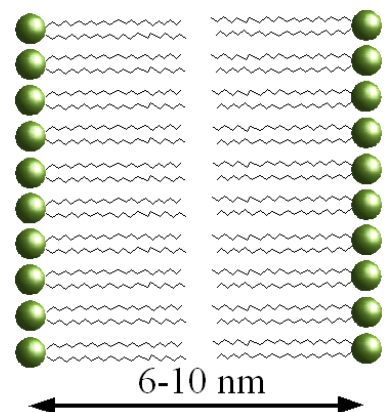
Fig. 4.1: Bicouche lipidique.
