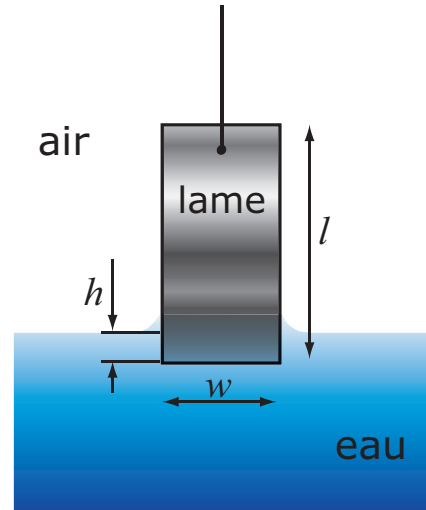
Fig. 4.6: La lame de Wilhelmy.
