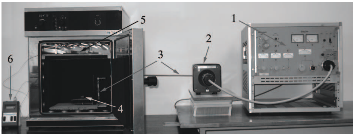
Fig. 8.8: Système d'exposition : (1) générateur haute tension Siemens RWON 14; (2) oscillateur à tube carinotron (Backward-Wave-Oscillator) Siemens RWO 75 (bande V) de puissance contrôlable ( P_{max} = 50 \text{ mW} à 60 GHz), (3) guides WR 15 (50-75 GHz), (4) antenne cornet pyramidal d'ouverture de dimensions 22.2 \times 16.7 \text{ mm}^2 , (5) plaque avec les cellules, (6) thermocouple.
