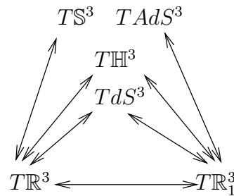
FIG. 4.8 – Les sept applications de Pogorelov infinitésimales.
