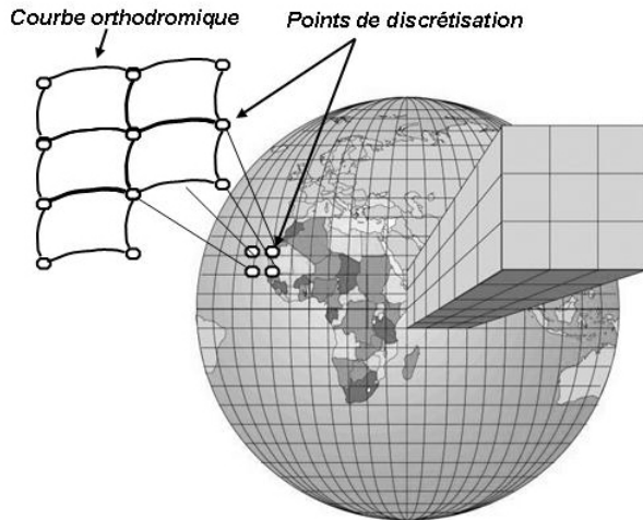
Figure III-2 : Maillage atmosphérique
