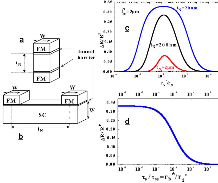
FIG. 1.3 – Structures émetteur ferromagnétique/canal semiconducteur/collecteur ferromagnétique dans les cas (a) d'une géométrie verticale et (b) d'une géométrie plane. (c) \Delta R/R_P de ces structures F/I/N/I/F (régime diffusif) en fonction du rapport r_b^*/r_N pour différentes longueurs de canal t_N . Les calculs sont effectués comme dans la Figure 1.2 avec F=Co et N=GaAs. (d) \Delta R/R_P de ces mêmes structures dans le cas d'un régime balistique en fonction du rapport entre le temps de séjour \tau_n et le temps de vie du spin \tau_{sf} dans le canal semiconducteur. D'après Fert et al. [31].
