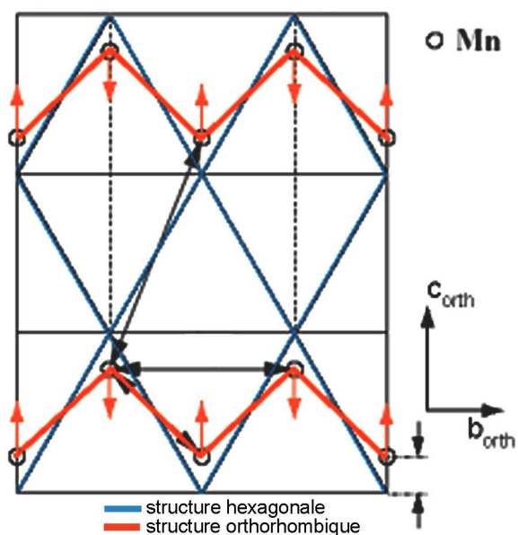
FIG. 3.2 – Représentation bidimensionnelle [selon (b_{\text{orth}}, c_{\text{orth}}) ] d'un plan de Mn dans la structure B31 [104]. Mise en évidence des déplacements des atomes de Mn (flèches) par rapport à leur position hexagonale pour former des chaînes en zig-zag.
