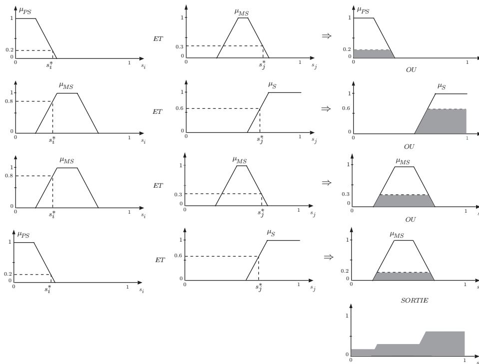
FIG. 3.13 – Exemple de combinaison des similarités s_i et s_j entre deux descripteurs i et j .
