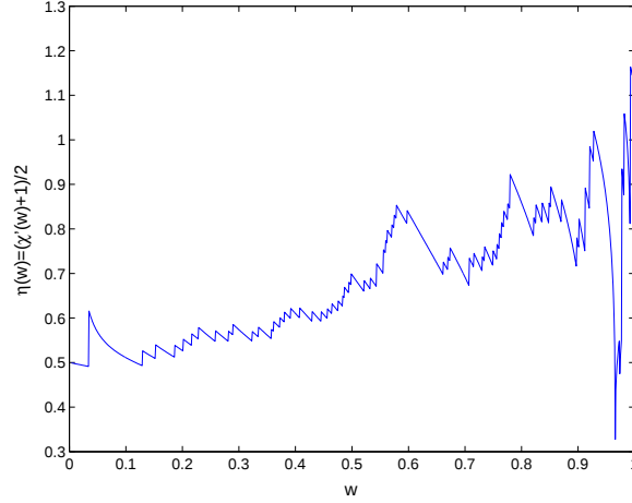
FIG. 8.5: Estimation de \eta , à partir de l'estimation de \bar{\chi}_1(w) : \eta(w) = \frac{\bar{\chi}_1(w)+1}{2} , sur les averses de Marseille supérieures à 13 mm.
