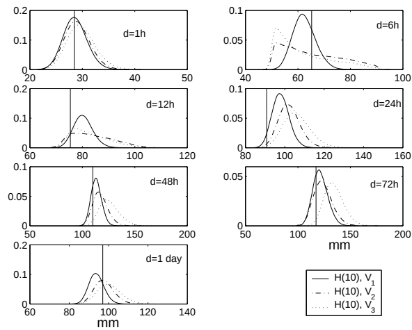
FIG. 4.9: Distributions a posteriori des quantiles H_d(10) pour d = 1 h, 6 h, 12 h, 24 h, 48 h, 72 h.
