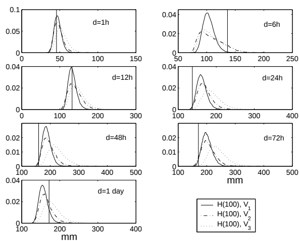
FIG. 4.10: Distributions a posteriori des quantiles H_d(100) pour d = 1 h, 6 h, 12 h, 24 h, 48 h, 72 h.
