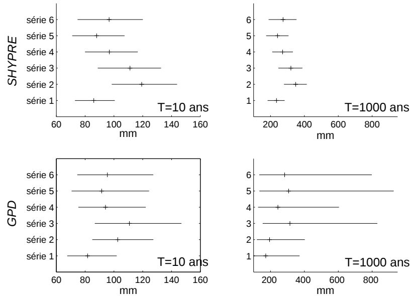
FIG. 6.5: Intervalles de confiance à 90% et médianes des estimations des quantiles de pluie journalière supérieure à 20 mm simulés par Shypre et estimés par la loi GPD, pour chaque sous-série. Les périodes de retour considérées sont 10 et 1000 ans.
