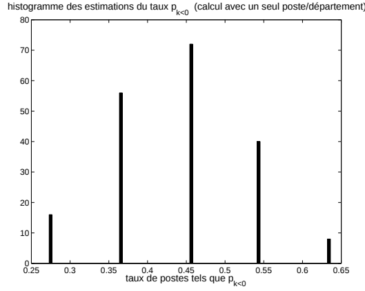
FIG. 3.2: Histogramme du taux p_{k<0} de postes tels que k < 0 , estimé sur les 192 échantillons de 11 séries appartenant à des départements français différents.
