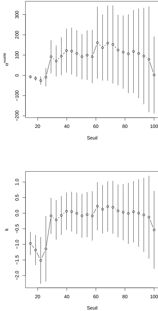
FIG. 7.4: Estimation des paramètres de la GPD en fonction du seuil pour la loi marginale de X_t , avec intervalle de confiance à 95%. Les graphes ont été tracés avec le package POT proposé par Ribatet (2006) sous le logiciel libre R. \alpha^{modifié}(w) = \alpha(w) + k(w)w avec \alpha(w), k(w) les paramètres de la GPD pour des données supérieures à w .
