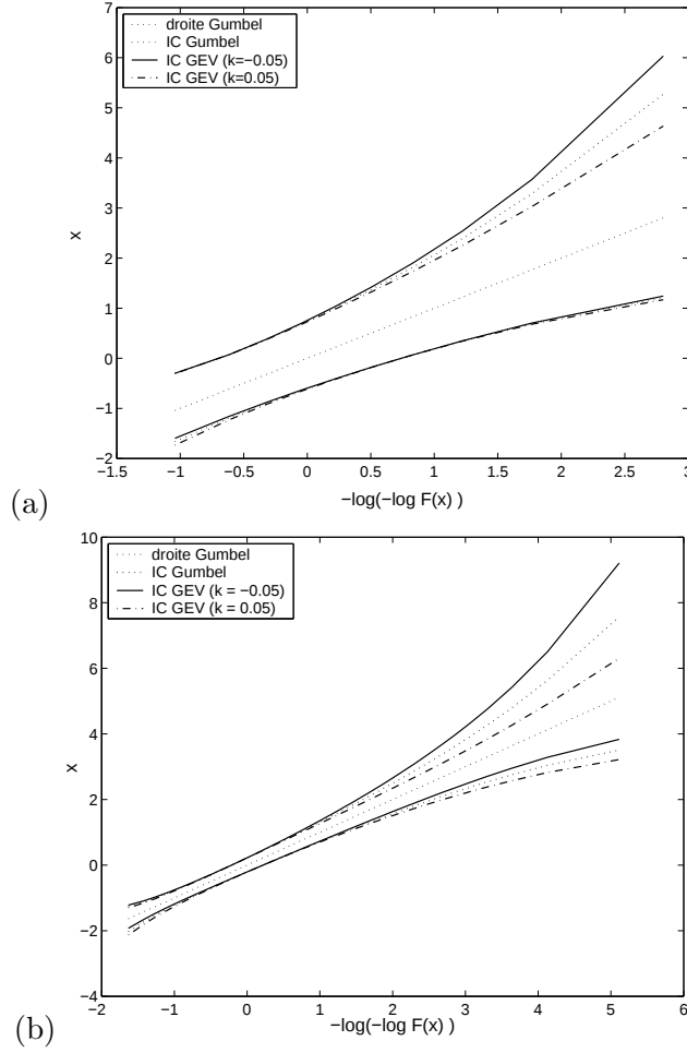
FIG. 2.2: Intervalles de confiance à 90% pour les statistiques d'ordre d'un échantillon de taille (a) n=10 , (b) n=100 , d'une population de loi GEV, pour différents paramètres de forme (Gumbel standard, GEV de paramètres \alpha = 1, \beta = 0, k = -0.05 , GEV de paramètres \alpha = 1, \beta = 0, k = 0.05 ).
