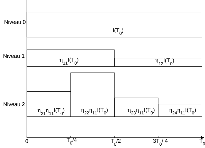
FIG. 5.4: Schéma descriptif de la construction d'une cascade multiplicative
