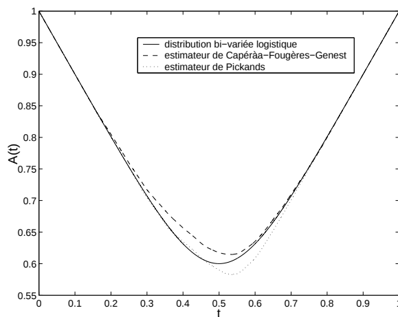
FIG. 4.6: Estimation de la fonction de dépendance de Pickands A(t) : comparaison entre des estimations non paramétriques de Pickands (1981), Pickands (1989), et Capéràa et al. (1997), et une estimation paramétrique (par maximum de vraisemblance) sous le modèle logistique.
