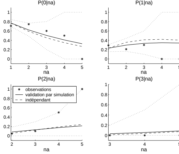
FIG. 8.11: Estimation des probabilités conditionnelles de dépassement du seuil u=25 mm p(j|na) . Les courbes en pointillés représentent les intervalles de crédibilité à 90% des probabilités p(j|na) sous hypothèse du modèle de persistance.
