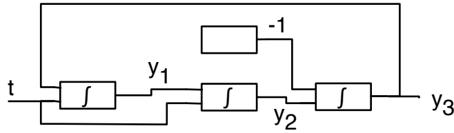
FIG. 1.9 – Génération de cos et sin par un GPAC. Sous forme de système d'équations, on a y_1' = y_3 , y_1(0) = 1 , y_2' = y_1 , y_2(0) = 0 , y_3' = -y_1 , y_3(0) = 0 . Il en suit que y_1 = \cos , y_2 = \sin , y_3 = -\sin .
