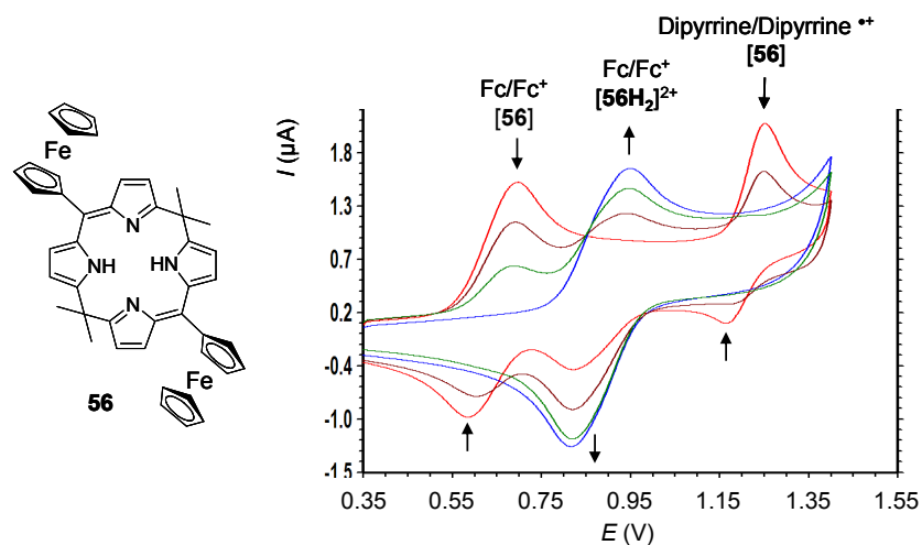
Figure II-39 : Evolution de la courbe de voltammétrie cyclique de 56 lors de l'ajout de \text{HClO}_4 (de 0 à 2 équivalents, 5 \cdot 10^{-4} M, \text{CH}_2\text{Cl}_2 0,1 M TBAP, électrode de travail : carbone vitreux \varnothing 3 mm, référence : \text{Ag}/\text{AgNO}_3 10^{-2} M).
