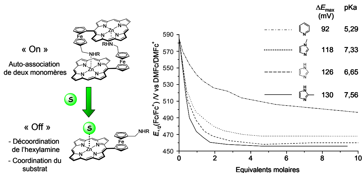
Figure III-66 : Titrage potentiométrique de 113Zn par la pyridine, l'imidazole, le 1-méthylimidazole et le 2-méthylimidazole ( \text{CH}_2\text{Cl}_2 0,1M TBAP, électrode de travail : disque de carbone \varnothing 3,5 mm, erreur : \pm 5 mV/s).
