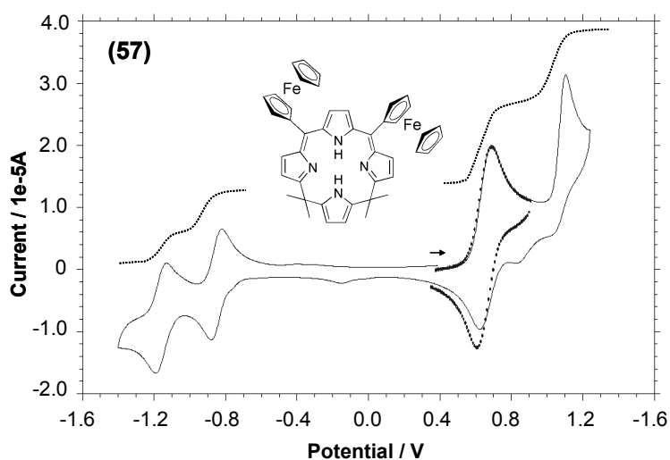
Figure II-26 : Courbes de voltammétrie cyclique et courbe de voltammétrie RDE de 57 enregistrées dans le dichlorométhane ( 5 \cdot 10^{-4} M, 0,1 M TBAP ; électrode de travail : disque de carbone vitreux \varnothing = 3 mm ; E vs. DMFc/DMFc + ; voltammétrie cyclique : \nu = 0,1 V/s ; RDE : \nu = 10 mV/s, vitesse de rotation de l'électrode 550 tours/min).
