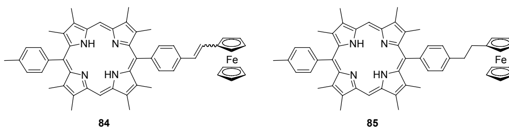
Figure III-9 : 5-ferrocénylvinylphényl-15-tolyle-2,3,7,8,12,13,17,18-octaméthylporphyrine 84 ; 5-ferrocényléthylphényl-15-tolyle-2,3,7,8,12,13,17,18-octaméthylporphyrine 85 [38].
