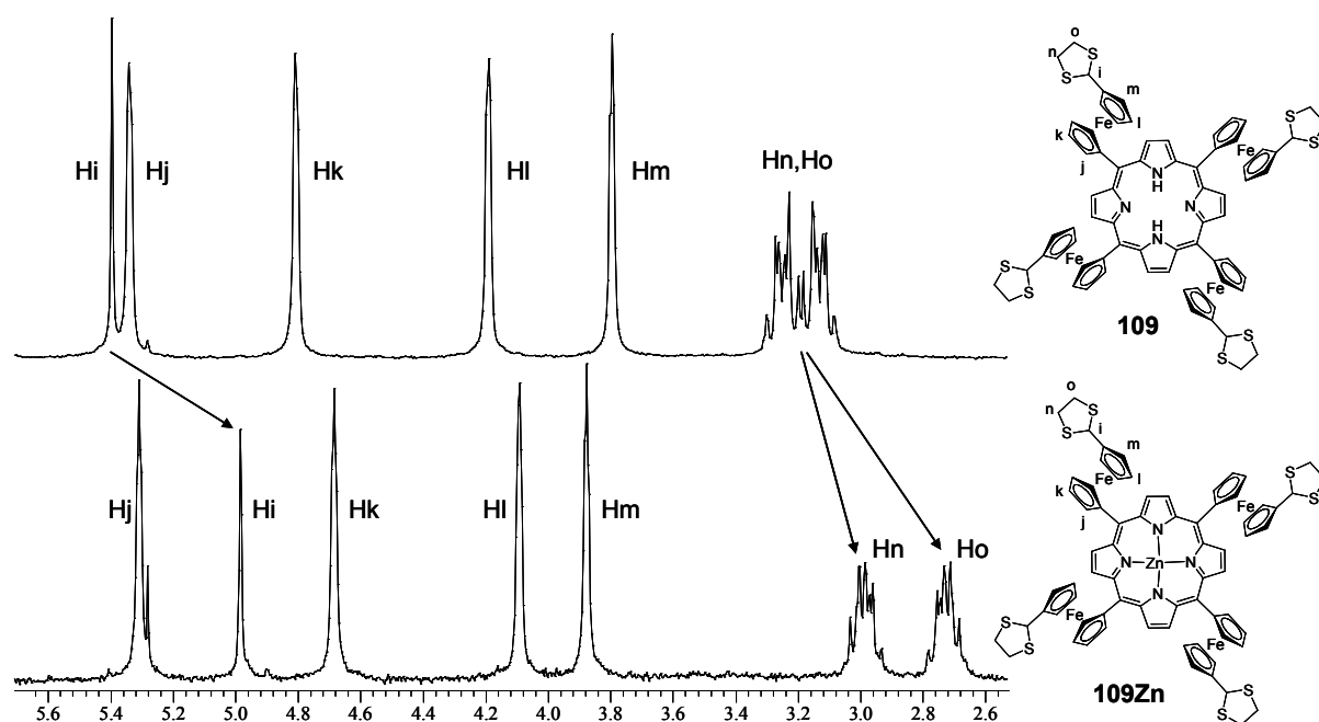
Figure III-29 : Spectre RMN ^1\text{H} partiel de 109 et 109Zn ( 5 \cdot 10^{-3} M, 250 MHz, \text{CDCl}_3 , 295 K).
