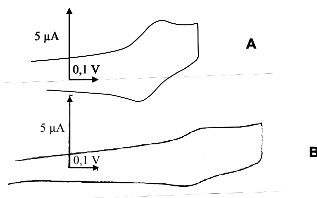
Figure III-45 : Courbes de voltammétrie cyclique partielles de 105 (A) avant et (B) après électrolyse à 1,26 V (2,1 équivalents d'électron, 10^{-4} M, \text{CH}_2\text{Cl}_2 0,25 M TBAP, électrode de travail : carbone vitreux Ø 3 mm, contre-électrode : fil de Pt, référence : AG/AgNO 3 10^{-2} M).
