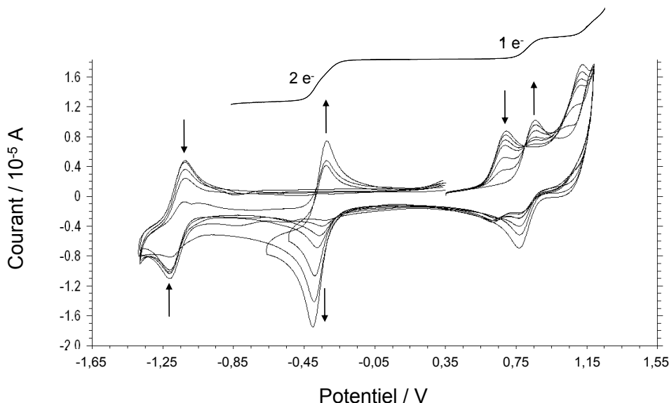
Figure III-46 : Evolution des courbes de voltammétrie cyclique lors de la protonation de 105 par \text{HClO}_4 (entre 0 et 2,5 équivalents molaires, 5 \cdot 10^{-4} M, \text{CH}_2\text{Cl}_2 0,1 M TBAP, \nu = 0,1 V/s, électrode de travail : disque de carbone vitreux \varnothing = 3 mm, contre-électrode : fil de Pt, référence : DMFC/DMFc + ). En haut, courbe de RDE enregistrée après l'ajout d'un excès d'acide perchlorique (2,5 équivalents molaires, \nu = 10 mV/s, vitesse de rotation : 550 tr/min).
