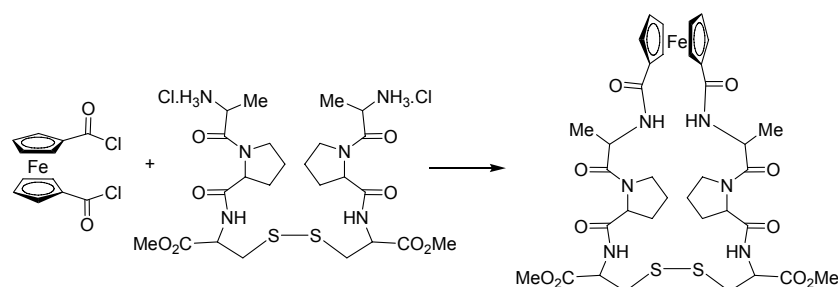
Figure IV-3 : Synthèse d'un pseudo-cyclopeptide rédox-actif pour la complexation réversible de cations métalliques [15].
