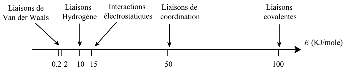
Figure I-9 : Energie de différentes interactions mises en jeu dans un processus de complexation.
