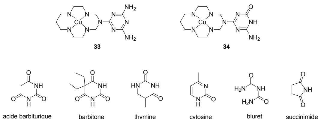
Figure I-33 : Récepteurs rédox pour la détection d'hétérocycles neutres [102].
