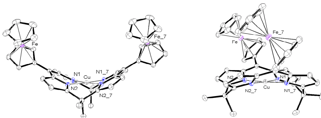
Figure II-14 : Vue ORTEP [55] de la calix[4]pyrines-(1.1.1.1) de cuivre (II) 56Cu . Les atomes d'hydrogène ne sont pas représentés pour des raisons de clarté. Les ellipsoïdes sont représentés au seuil de probabilité de 45%.
