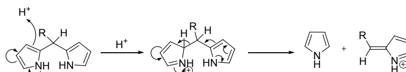
Figure III-24 : Mécanisme de décomposition du dipyrrométhane en milieu acide.
