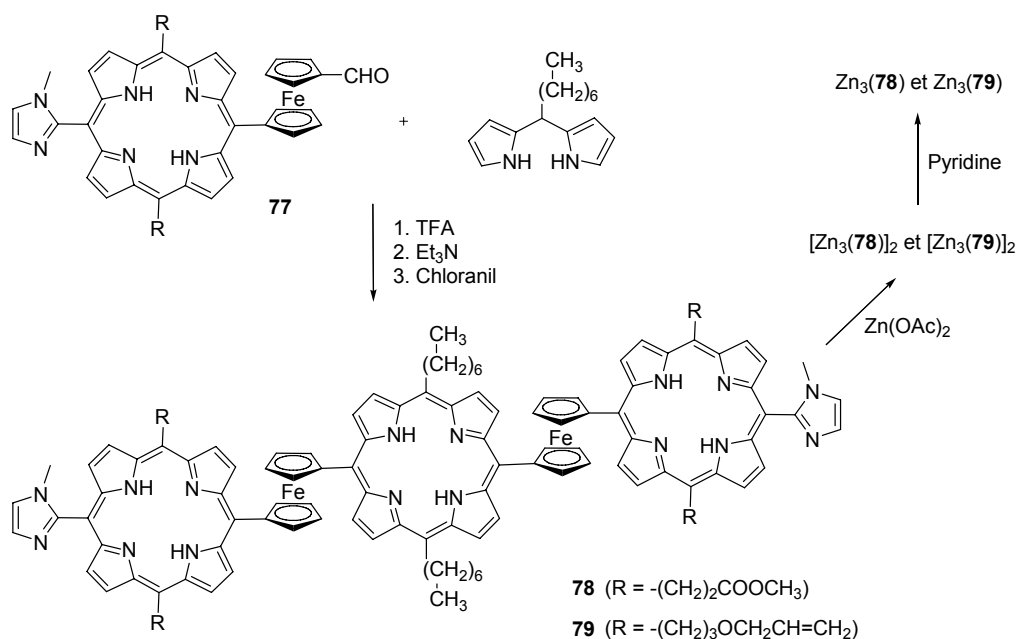
Figure III-6 : Schéma de synthèse de la 5,15-bis[1'-(15''-(1-méthylimidazol-2-yl)-10''',20''-bis(2-méthoxycarbonyléthyl)porphyrine-5''-yl]ferrocényl]-10,20-bis( n -heptyl)porphyrine 78 et de la 5,15-bis[1'-(5'',15''-bis(3-allyloxypropyl)-10''-(1-méthylimidazol-2-yl)porphyrine-20''-yl]ferrocényl]-10,20-bis( n -heptyl)porphyrine 79 [27].
