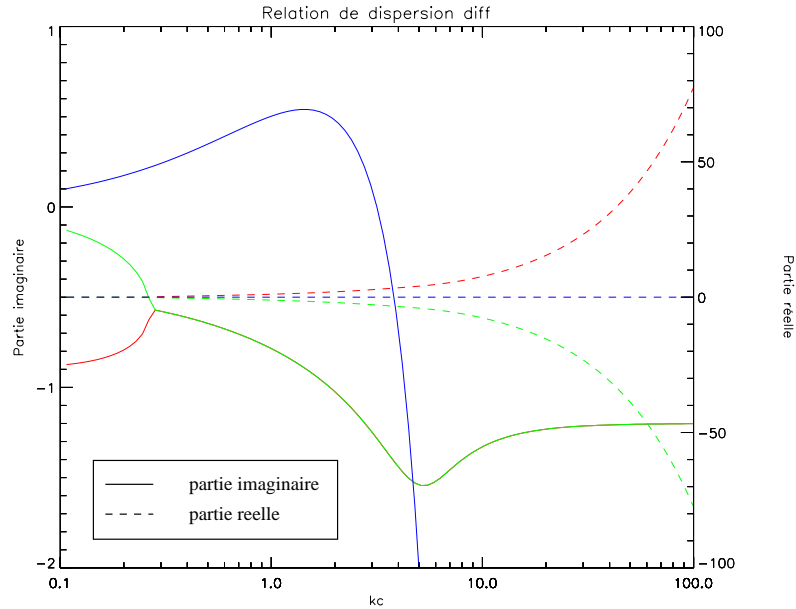
FIG. 5.17 – Relation de dispersion avec une longueur de diffusion \lambda = c/(10\omega_\rho) qui correspond donc à kc = 10\omega_\rho . On se place à n_H = 5/\text{cm}^3 , et à l'équilibre thermo-chimique. Toutes les unités sont normalisées par \omega_\rho .
