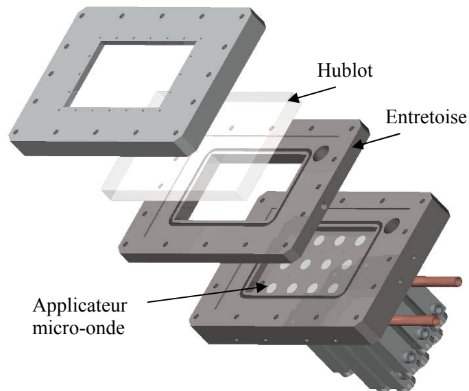
Figure 2.2. Vue éclatée du réacteur.
