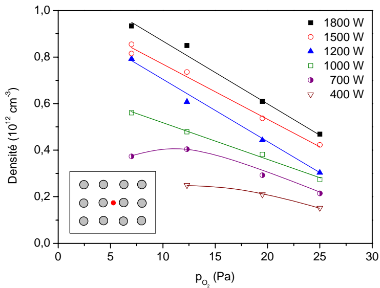
Figure 6.5. Densité du plasma en fonction de la pression d'oxygène pour plusieurs puissances micro-onde.
