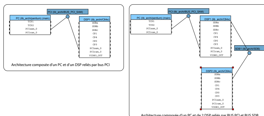
FIG. 6.7 – Architectures pour le portage des applications LAR
