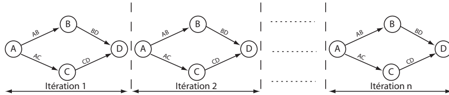
FIG. 2.1 – Graphe de dépendance sur n itérations
