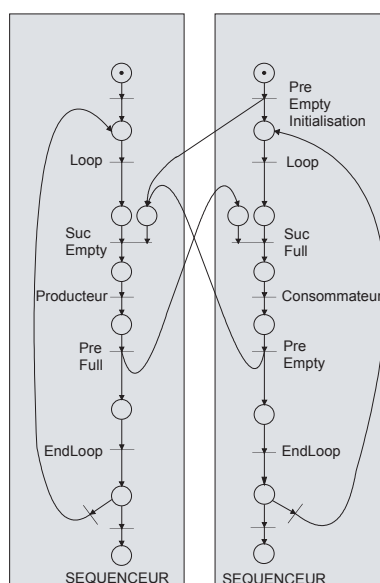
FIG. 2.18 – Réseau de Petri avec le maximum de parallélisme
