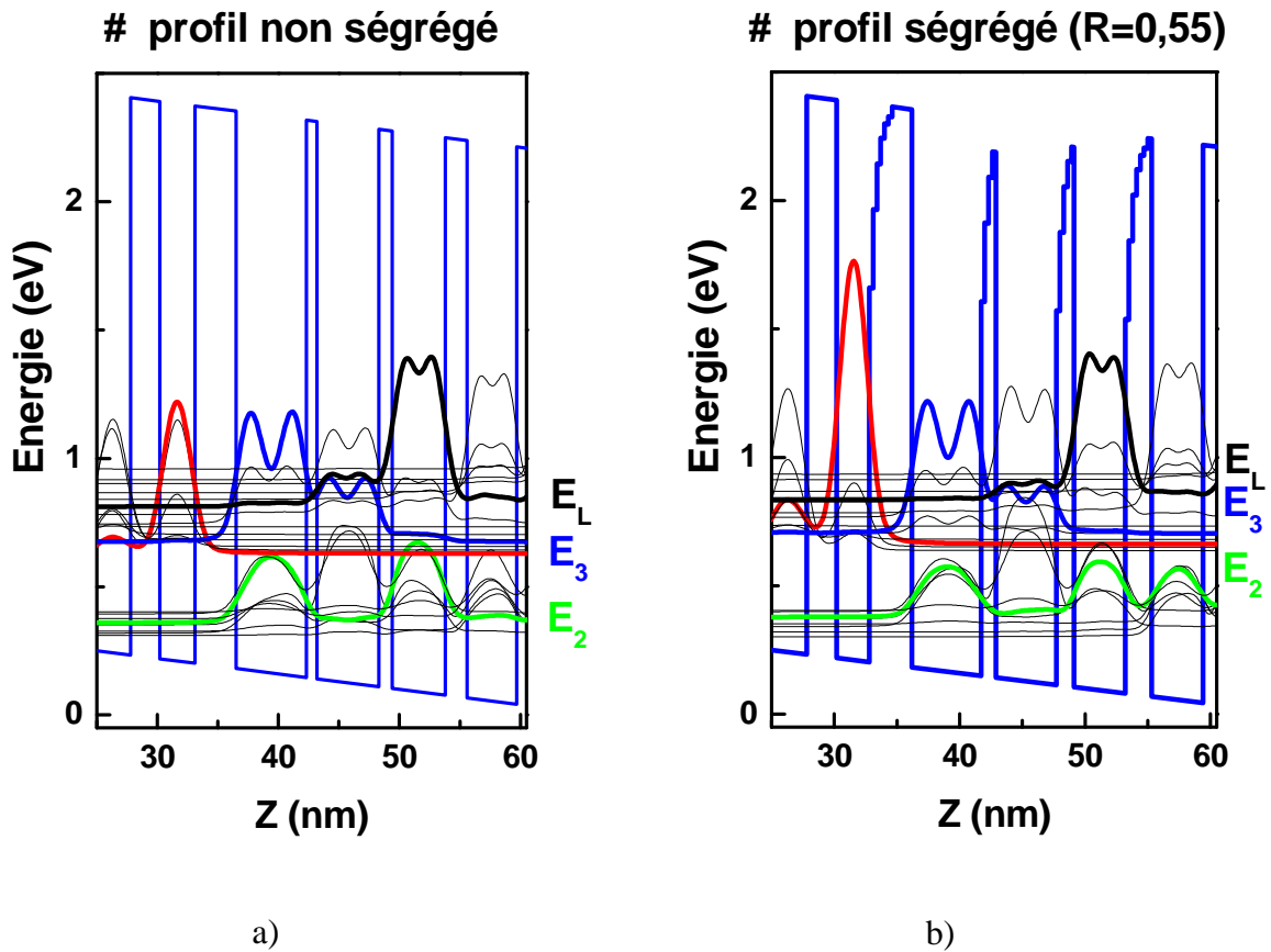
Figure 5.26: Diagramme de bande de conduction de la zone active du laser à cascade quantique InAs/AlSb étudié à la figure 5.25 sous champ électrique ( V = 60 \text{ kV/cm} ). La structure est calculée a) sans ségrégation d'In et b) en tenant compte de la ségrégation de l'In.
