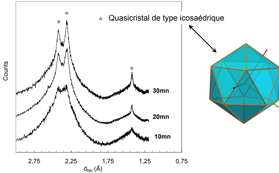
Fig. A.5 : Diagramme de diffraction X pour les échantillons traités à 410°C moins de 30mn. L'unique type de cristaux qui est indexé correspond à un quasicristal de type icosaédrique (comme représenté).
