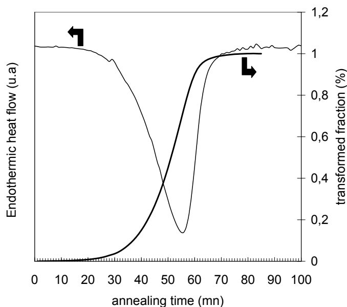
Fig. I.10 : Analyse de la cristallisation par DSC isotherme dans le cas d'un alliage base Mg (tiré de [Puech et al., 2006]). La courbe de cristallisation obtenue en DSC isotherme ainsi que la fraction transformée issue de l'intégrale de cette courbe sont représentées.
