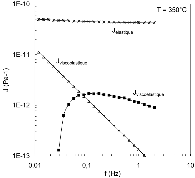
Fig. C.1 : Calcul des composantes élastiques, viscoélastiques et viscoplastiques issues d'un essai de spectromécanique sur un échantillon de Vit 1 amorphe à une température de 350°C.
