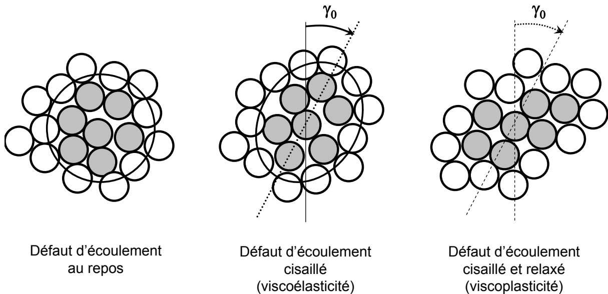
Fig. IV.12 : Évolution d'un défaut d'écoulement passant d'un état au repos vers un état cisailé (correspondant à une déformation viscoélastique) puis vers un état relaxé (correspondant à une déformation viscoplastique).
