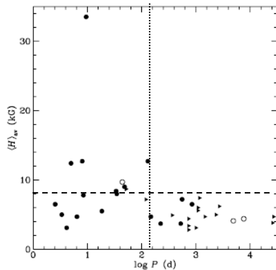
FIG. 2.3: Module du champ magnétique moyen, moyenné sur une période, en fonction de la période des étoiles Ap/Bp. Les ronds représentent les périodes déterminées précisément et les triangles représentent les étoiles dont seule une limite inférieure a pu être mesurée (Mathys et al. 1997).
