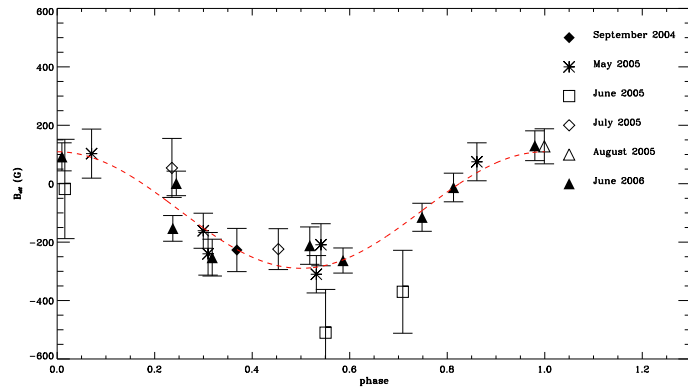
FIG. 13.18: B_\ell en fonction de la phase pour HD 200775. La ligne en tirets est le meilleur ajustement sinusoidal.
