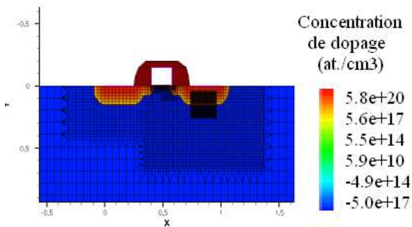
Figure III - 16 : Présentation de la structure simulée : NMOS de technologie 0,18 \mu\text{m} . Le simulateur composant utilisé est dessis de ISE de la société Synopnys. Le quadrillage représente la structure de maillage.
