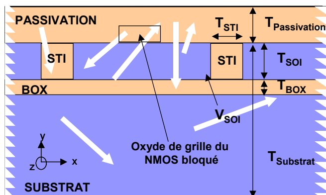
Figure IV - 3 : Modélisation MC-DASIE pour les technologies SOI. V_{SOI} le volume de SOI (body+LDD), T_{Passivation} l'épaisseur de passivation, T_{Substrat} , l'épaisseur de substrat, T_{SOI} la couche de passivation, T_{BOX} l'épaisseur de la BOX et T_{STI} l'épaisseur des STI (autour de V_{SOI} ). Les flèches blanches représentent les parcours des ions. Le substrat et le volume de SOI sont modélisés avec des atomes de Si. La passivation, STI et BOX sont en oxyde de silicium et peuvent être modélisés avec à la fois des atomes de Si et de O ( SiO_2 ) ou seulement les atomes de Si (comme du Silicium).
