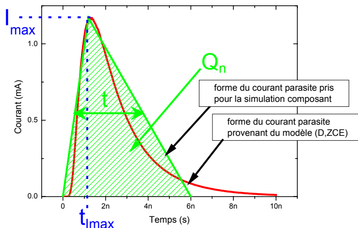
Figure IV - 14 : Illustration du courant parasite et des paramètres I_{max} , t_{imax} , Q_n et t
