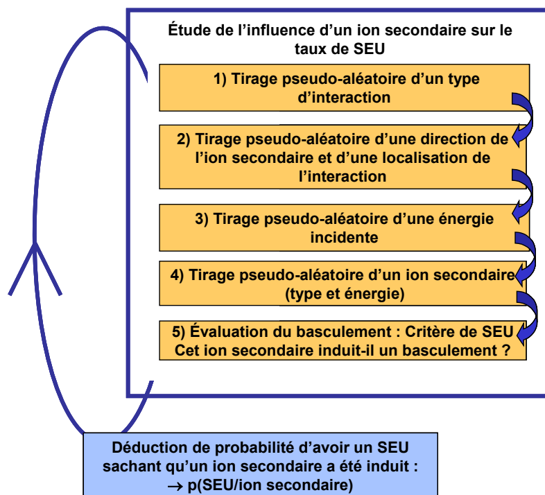
Figure IV - 32 : Etapes du calcul Monte-Carlo de p(\text{SEU}/\text{ion secondaire})
