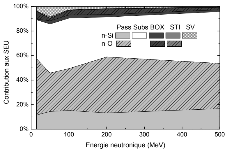
Figure V - 22 : Répartition des types d'interaction, qui induisent des SEU pour le composant SOI 0.2 μm sans BT en fonction de l'énergie neutronique.
