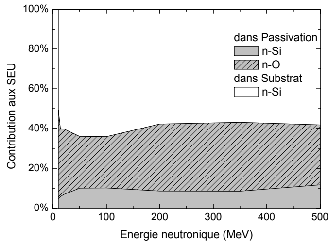
Figure V - 21 : Répartition des types d'interaction, qui induisent des SEU pour le composant bulk 0,25 μm en fonction de l'énergie neutronique.
