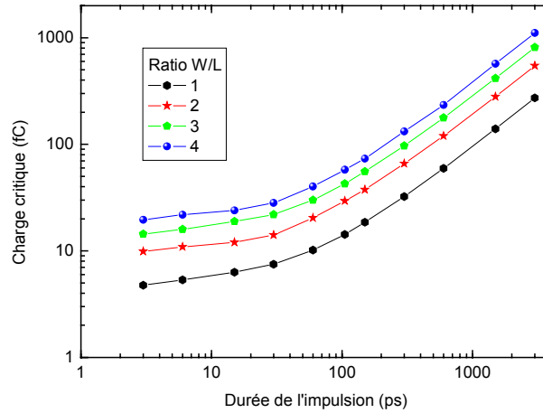
Figure IV - 28 : Charge critique d'une technologie Bulk 0,25 \mu\text{m} en fonction de la durée de l'impulsion pour différentes largeurs de grille.
