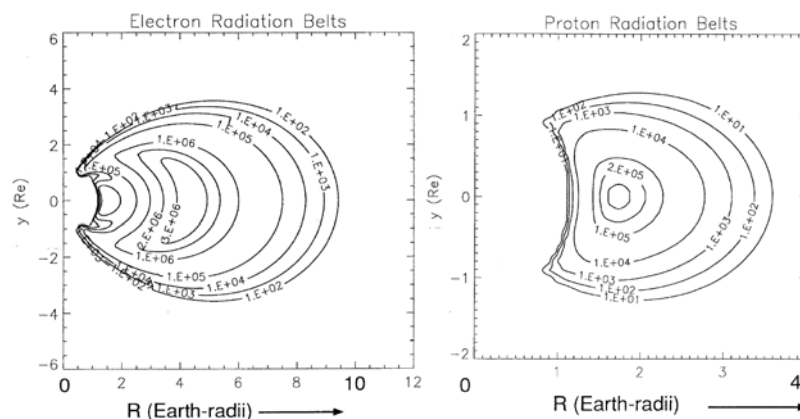
Figure I - 9 : Iso flux ( \text{cm}^2 \cdot \text{s}^{-1} ) des ceintures de radiation des électrons et des protons en coordonnées cylindriques par rapport à l'axe du dipôle magnétique terrestre en unité de rayon terrestre d'après les travaux de E. J. Daly [ESA - 1993]
