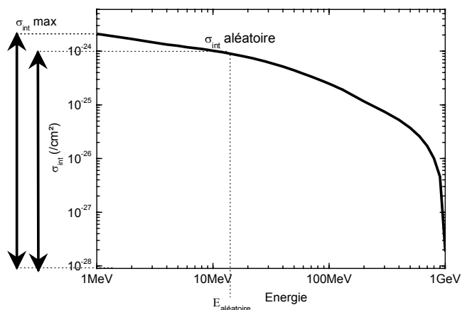
Figure IV - 40 : Intégrale du produit de la section efficace de production avec la distribution énergétique normalisée du spectre neutronique terrestre en fonction de l'énergie incidente : \sigma_{int}(E)
