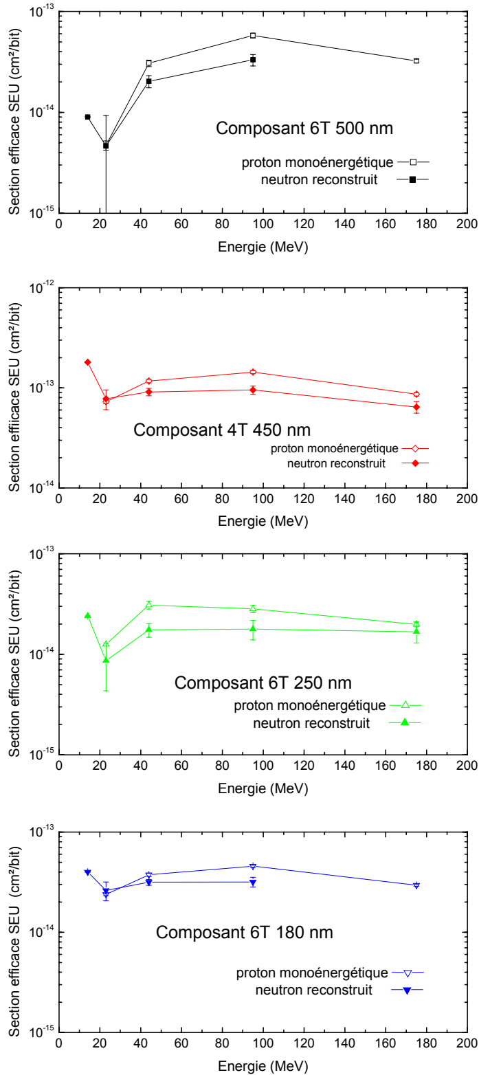
Figure V - 15 : Sections efficaces SEU en fonction de l'énergie. Les données protoniques sont expérimentales. Les données neutroniques sont expérimentales et corrigées avec les valeurs C_{TAILMCD} . [JESD - 2001].
