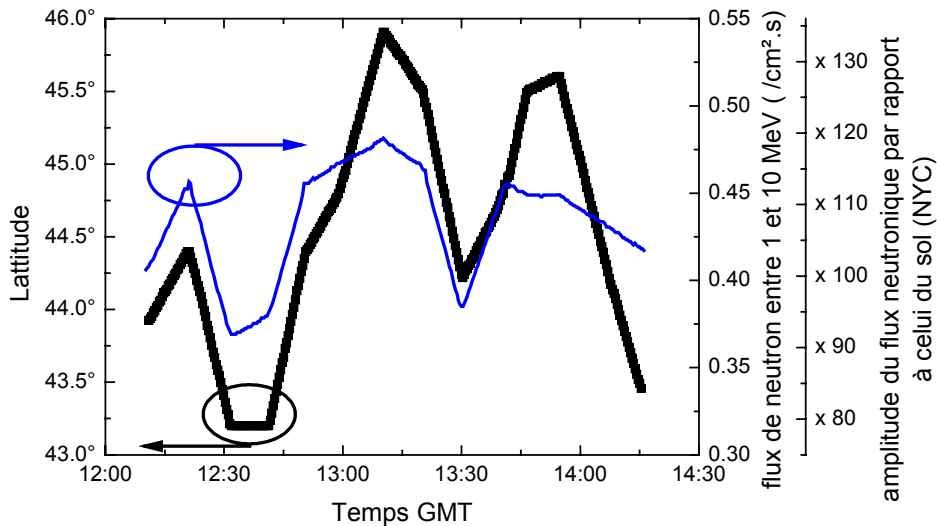
Figure I - 17 : Variations de la latitude et du flux de neutrons 1 à 10 MeV lors d'un vol avionique à une altitude de 10.6 km [Hubert - 2004].
