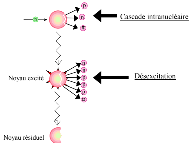
Figure II - 15 : Représentation schématique de processus d'interaction neutron-matière traité par HETC.
