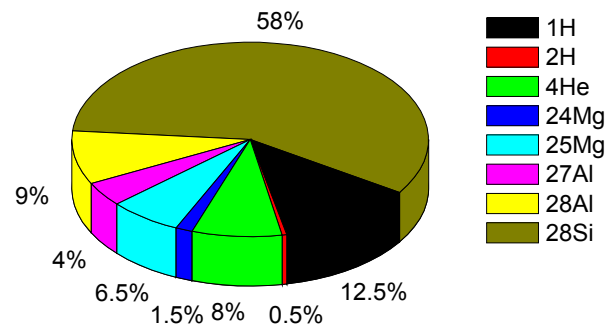
Figure IV - 42 : Répartition des sections efficaces de production des ions secondaires de l'interaction neutron-atome de silicium ( E_n = 14 \text{ MeV} ).
