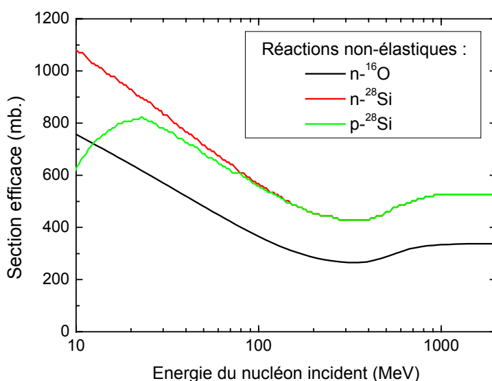
Figure II - 16 : Section efficace d'interaction non-élastique de n\text{-}^{16}\text{O} , n\text{-}^{28}\text{Si} et p\text{-}^{28}\text{Si} d'après un modèle de Glauber amélioré [Duarte - 2004].
