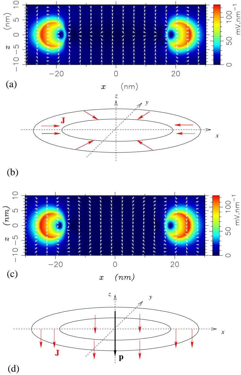
FIG. 5.9 – (a) Distribution du champ électrique du mode pair M = 0, N = 0 ( \omega_{M=0, N=0; \Pi=1}^+ / c ) dans le plan xz : l'intégration sur l'objet d'une telle distribution donne des moments dipolaires électrique et magnétique nuls (b). Distribution du champ électrique du mode impair M = 0, N = 1 ( \omega_{M=0, N=1; \Pi=1}^- / c ) dans le plan xz (c) : les composantes du champ selon l'axe z se s'annulent pas lors de l'intégration, il en résulte un moment dipolaire électrique non nul (d).
