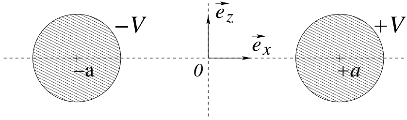
FIG. 2.1 – Construction des coordonnées bipolaires : ce système de coordonnées est construit à partir du problème de deux cylindres portés à des potentiels égaux en valeur absolue et de signes opposés, placés en -a et +a .
