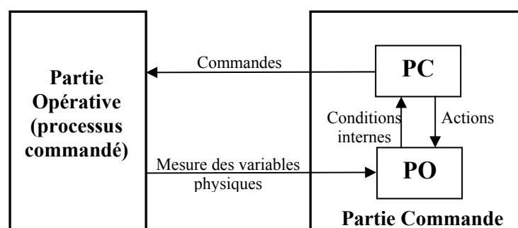
Figure 14 : Décomposition du système en PC et PO
