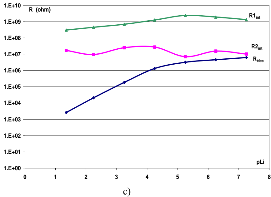
Figure 2.87 : a) valeur des impédances Q en fonction de la concentration b) valeur des coefficients n en fonction de la concentration c) valeur des résistances R en fonction de la concentration
