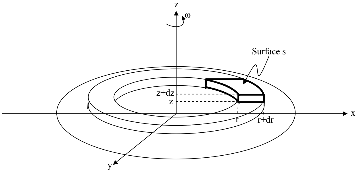
Figure 2.50 : Anneau élémentaire de polymère
