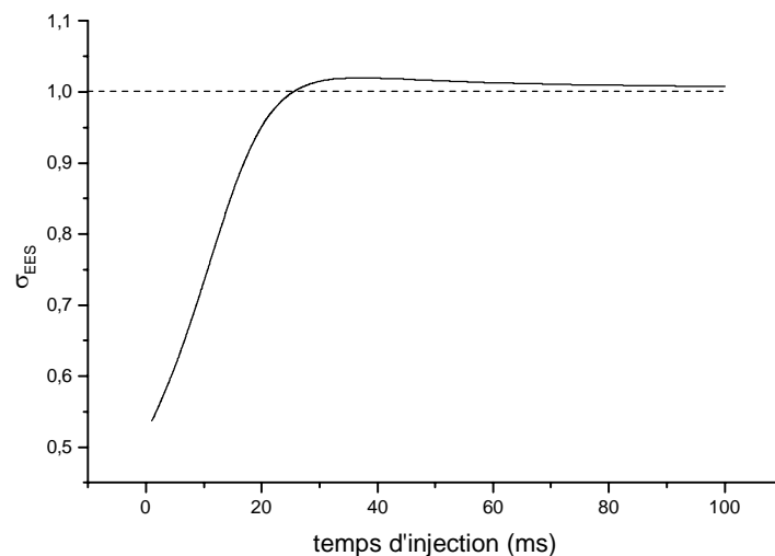
Figure 12: évolution du rendement d'émission électronique (Alumine, E_0 = 30 \text{ keV} ; J_0 = 10^{-5} \text{ A/cm}^2 ; pas de pièges à électrons)
