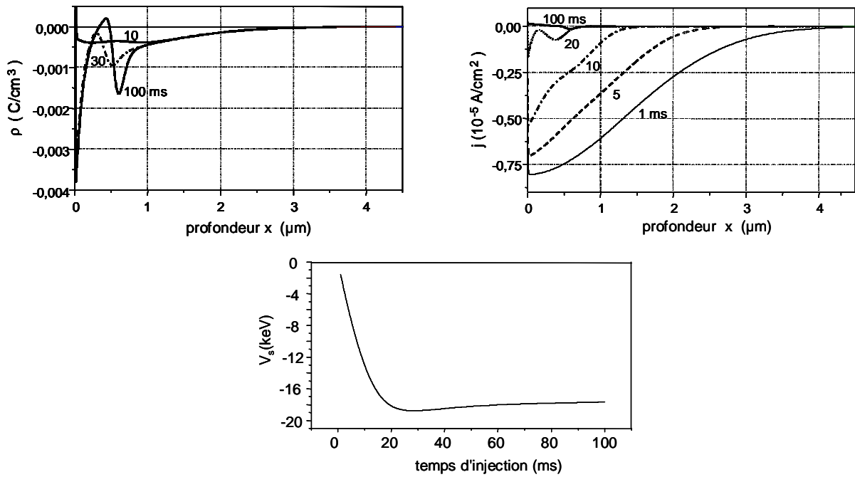
Figure 11: Evolutions de la densité totale de charges, du courant total et du potentiel de surface en fonction de la profondeur et (ou) du temps. (Alumine, E_0 = 30 \text{ keV} ; J_0 = 10^{-5} \text{ A/cm}^2 ; pas de pièges à électrons)
