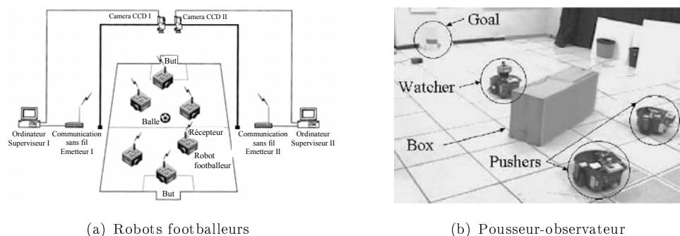
FIG. 2.1 – Tâches coopératives contrôlées d’une manière centralisée
