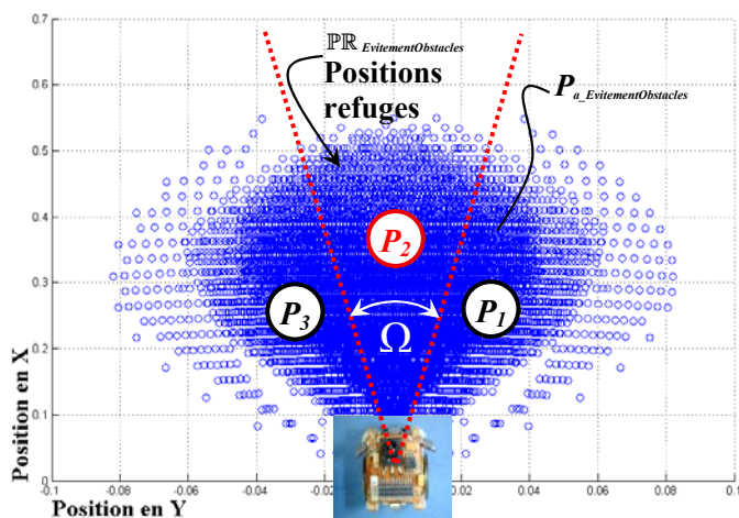
FIG. 4.8 – Positions atteignables " P_a_{\text{ÉvitementObstacles}} " et positions refuges " \mathbb{P}R_{\text{ÉvitementObstacles}} " du comportement d' évitement d'obstacles .
