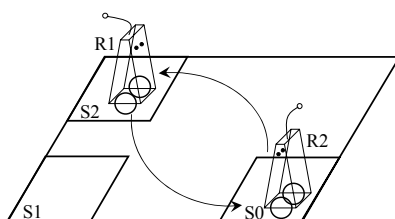
FIG. 2.3 – Situation d'interblocage
