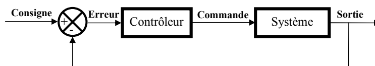
FIG. 1.3 – Schéma d’un asservissement conventionnel
