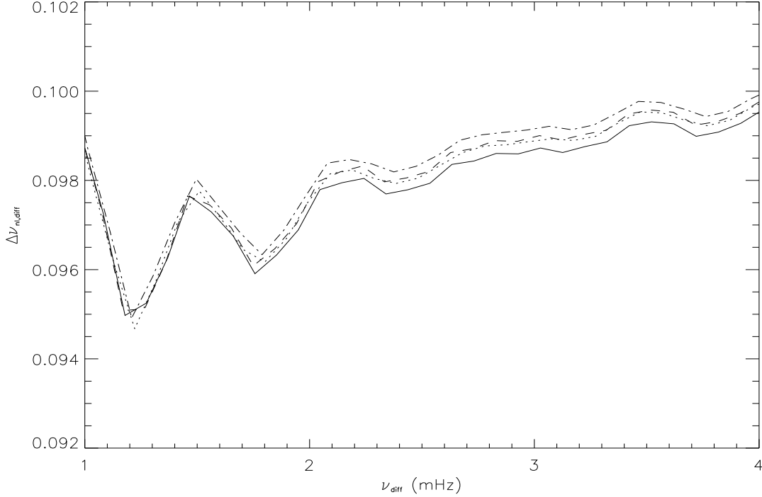
FIG. 2.2: Grandes séparations \Delta\nu_{n,l} pour l = 0 (trait continu), l = 1 (tirets), l = 2 (pointillés) et l = 3 (trait-points) pour un modèle standard de 1.2 M_{\odot} à 3.3 Gyrs.
