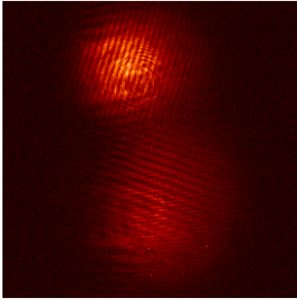
FIG. 6.6 – Figure de diffraction obtenue par focalisation de la pupille de sortie sur un détecteur. Ici, le collage à été arrêté à 7 fibres, car un décalage manifeste des fibres a été détecté, séparant les différents faisceaux sur deux taches Gaussienne distinctes. On peut cependant noter la très bonne cohérence de la lumière.
