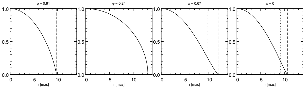
FIG. 3.12 – Profils d’assombrissement de \chi Cyg aux différentes phases stellaires ( I(r) = (1 - (2r/\theta_*)^2)^{\alpha/2} ). En pointillées les valeurs du diamètre de Rosseland. En tirets, les valeurs de \theta_*/2 .
