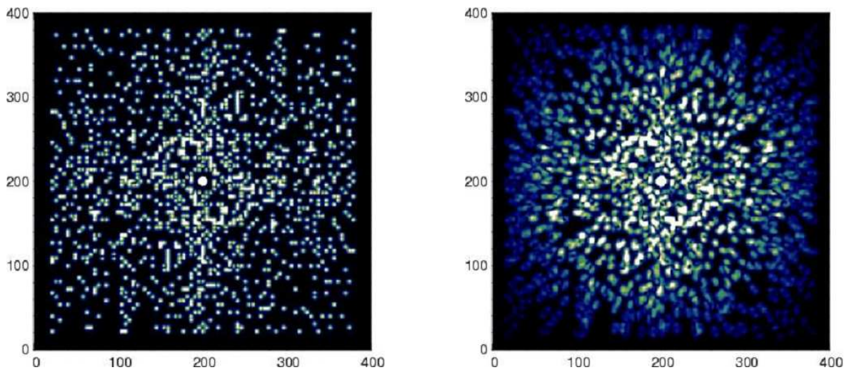
FIG. 5.15 – Effet du chromatisme sur le plan des fréquences spatiales. A gauche, les pics franges sont nettement définis sur l'image achromatique. A droite : le chromatisme ( 620 \text{ nm} < \lambda < 640 \text{ nm} ) disperse les pics franges sur plusieurs fréquences spatiales.
