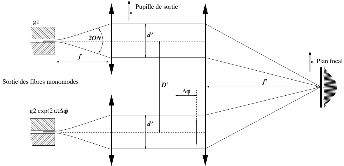
FIG. 5.6 – Schéma d'un système de recombinaison à deux faisceaux
