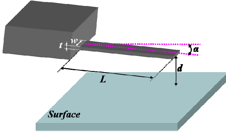
Figure 3 : Poutre encastree-libre de longueur L , de largeur w , d'épaisseur t inclinée d'un angle \alpha par rapport à l'horizontal et à une distance d de la surface à imager.
