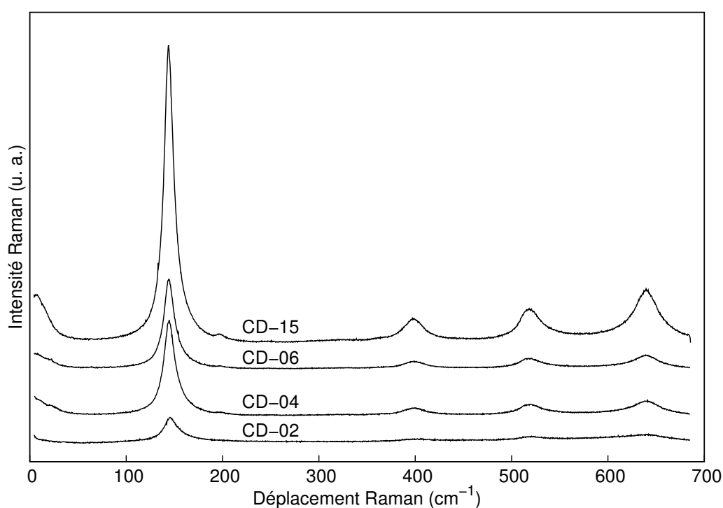
FIG. 2.9 – Spectres Raman des poudres de \text{TiO}_2 « chimie douce » traitées thermiquement à 300^\circ\text{C} sous flux d'air reconstitué ( 0,2\text{L}/\text{min} ) pendant 2, 4, 6, 15 heures (de bas en haut). La rampe de température est de 2^\circ\text{C}/\text{min} .
