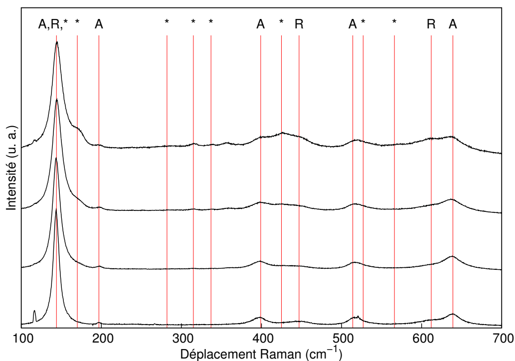
FIG. 2.2 – Spectres Raman des poudres de \text{TiO}_2 Degussa P25 broyées pendant 0, 5, 15 et 30 minutes (de bas en haut). A : Anatase, R : Rutile et * : \text{TiO}_2 II
