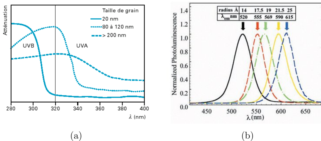
FIG. 1 – (a) Limite d'absorption UV de \text{TiO}_2 en fonction de la taille des grains [1]. (b) Photoluminescence de cœur/couronne CdSe/ZnS pour une longueur d'onde d'excitation de 350 nm [2].
