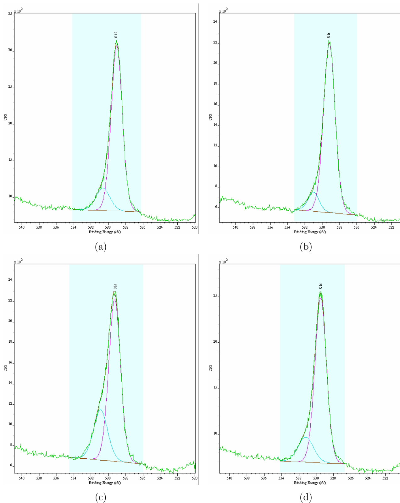
FIG. 4.7 – Spectres XPS du pic O 1s des poudres de \text{TiO}_2 synthétisées : (a) par précipitation à partir de l'isopropoxyde de titane puis traitée 15 heures sous flux d'air reconstitué : CD-15, (b) par microémulsion inverse ME-1T, par synthèse hydrothermale en continu (c) HT-6 et (d) HT-7. (Appareil utilisé : AES-ESCA-ELS-MAG2, K_\alpha Al, résolution 1,2 eV, LRRS)
