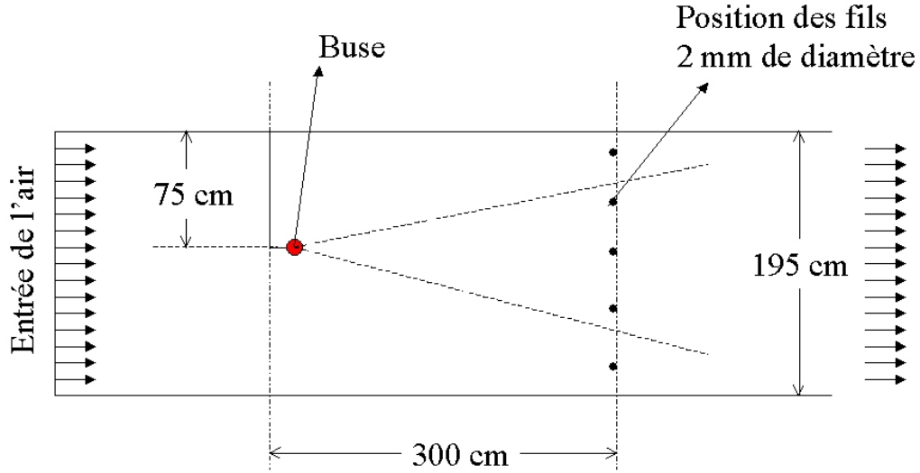
FIG. 3.3 – Configuration des essais dans la soufflerie
