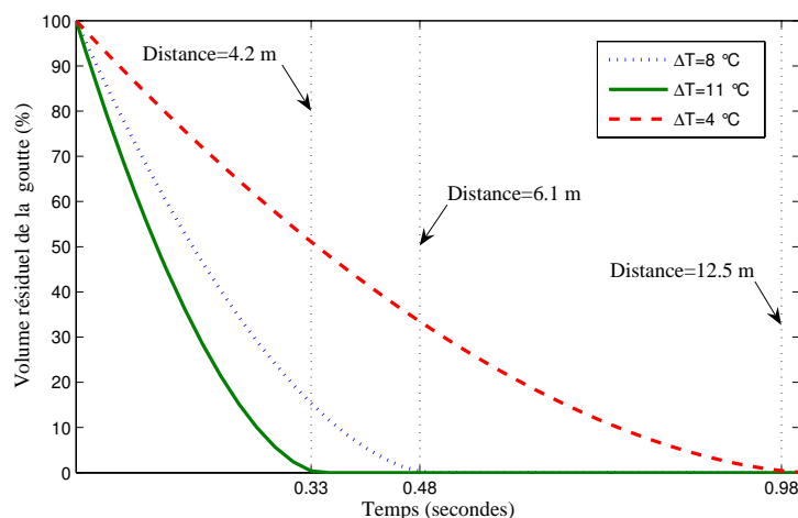
FIG. 3.9 – Variation de volume d'une goutte d'un diamètre initial de 28 \mu\text{m} pour plusieurs différences psychrométriques ( \Delta T ). Distance parcourue par la goutte avant évaporation totale pour une vitesse d'éjection initiale de 12.8 \text{ m}\cdot\text{s}^{-1}
